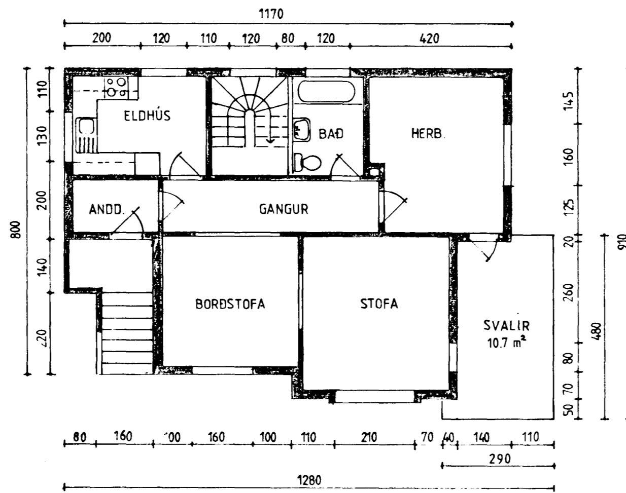
GRUNNMYND I. HÆÐ Mkv. 1:100
