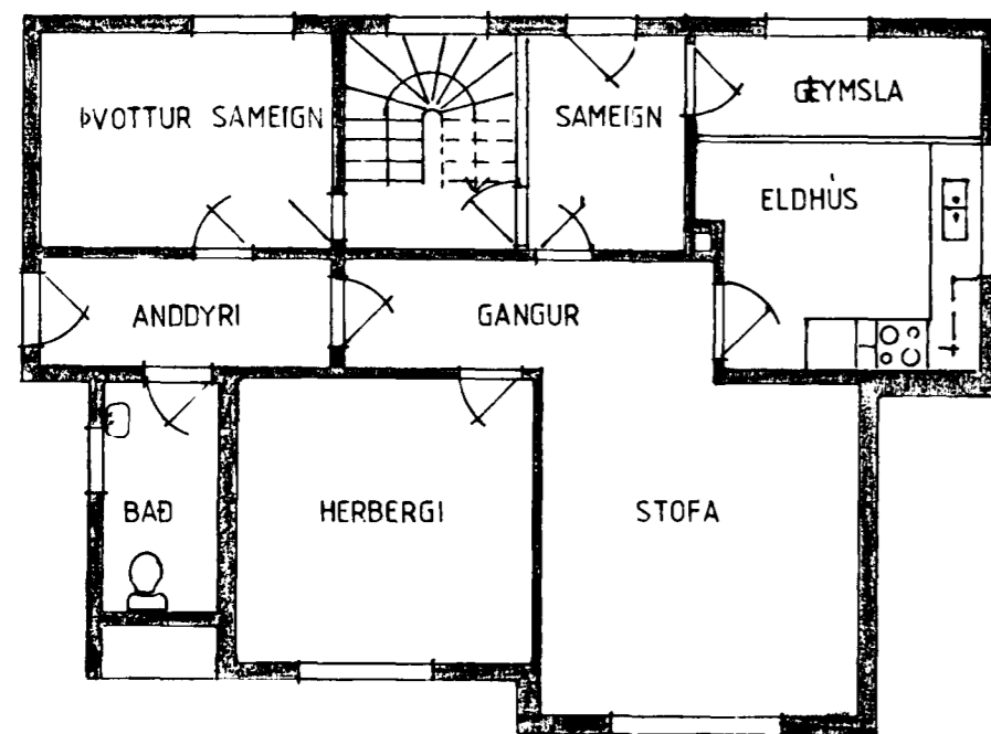
GRUNNMYND KJALLARI Mkv. 1:100
