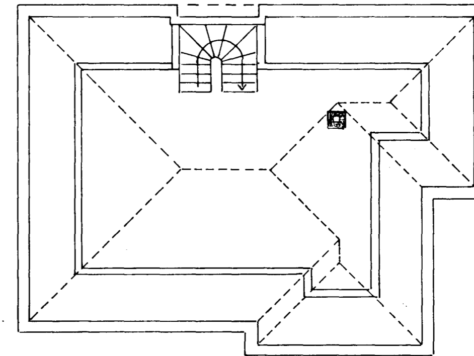
GRUNNMYND RISHÆÐAR Mkv. 1:100
