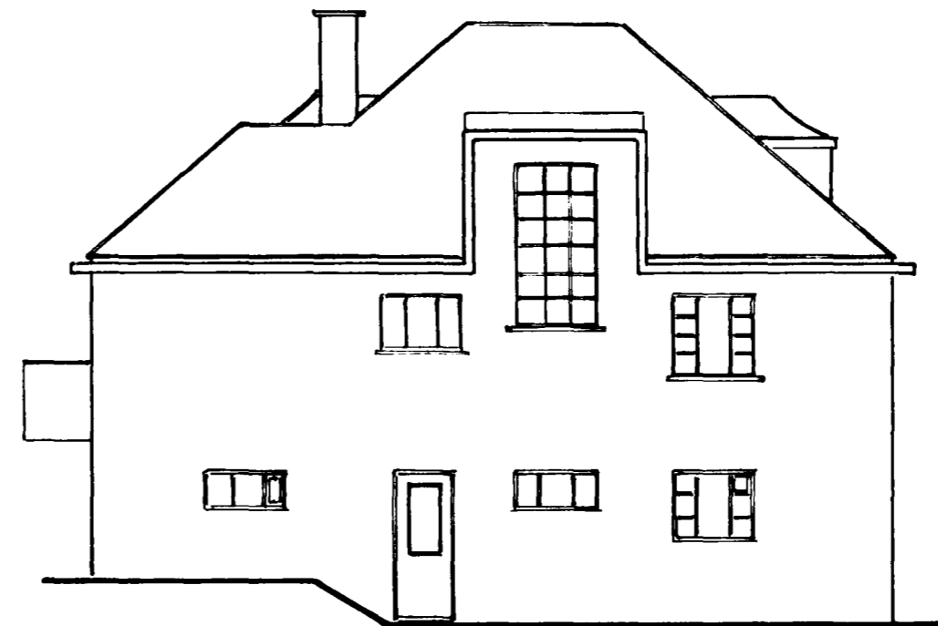
NORDAUSTURHLID Mkv. 1:100
