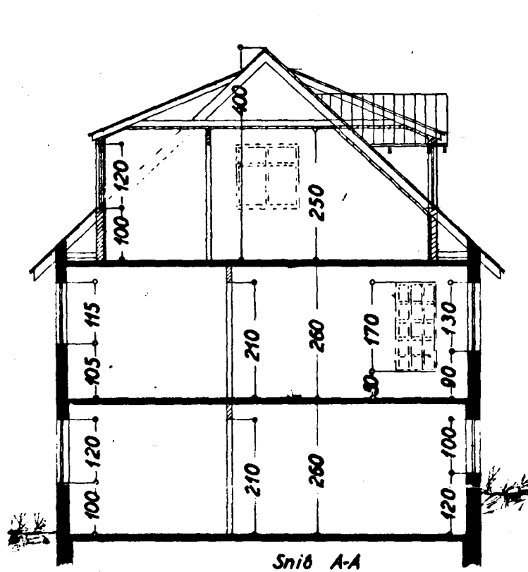
Snið A-A
