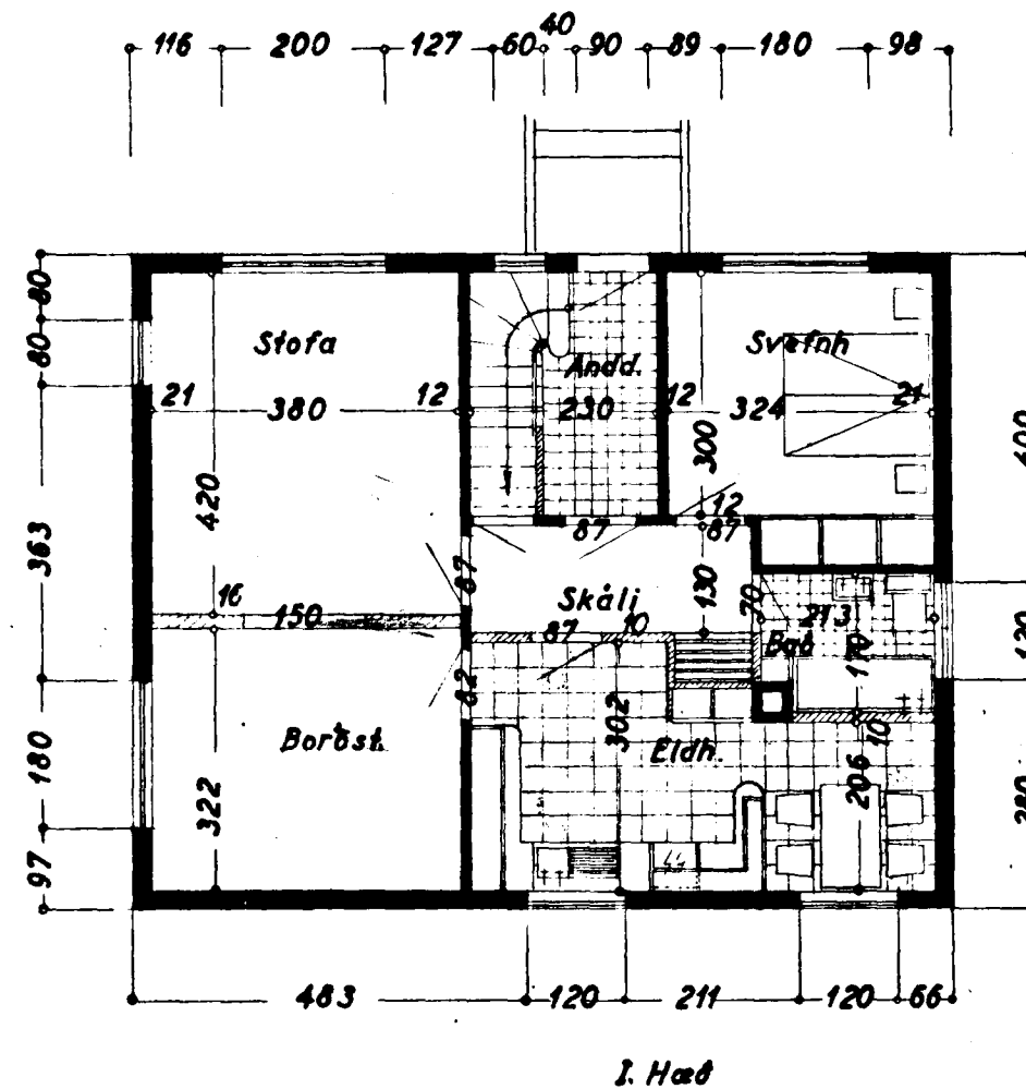
1. Hæð
