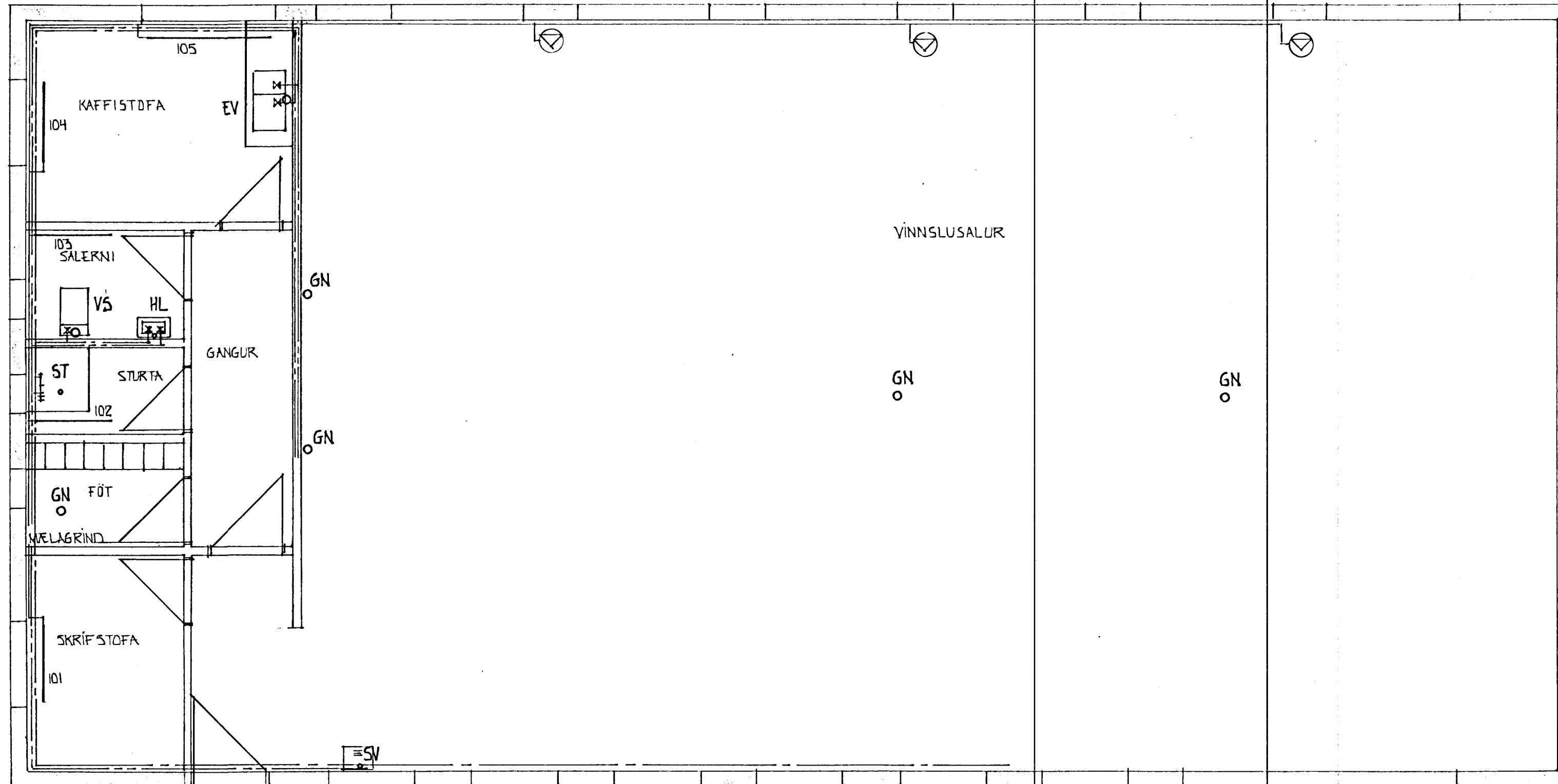
GRUNNMYND M 1:50
