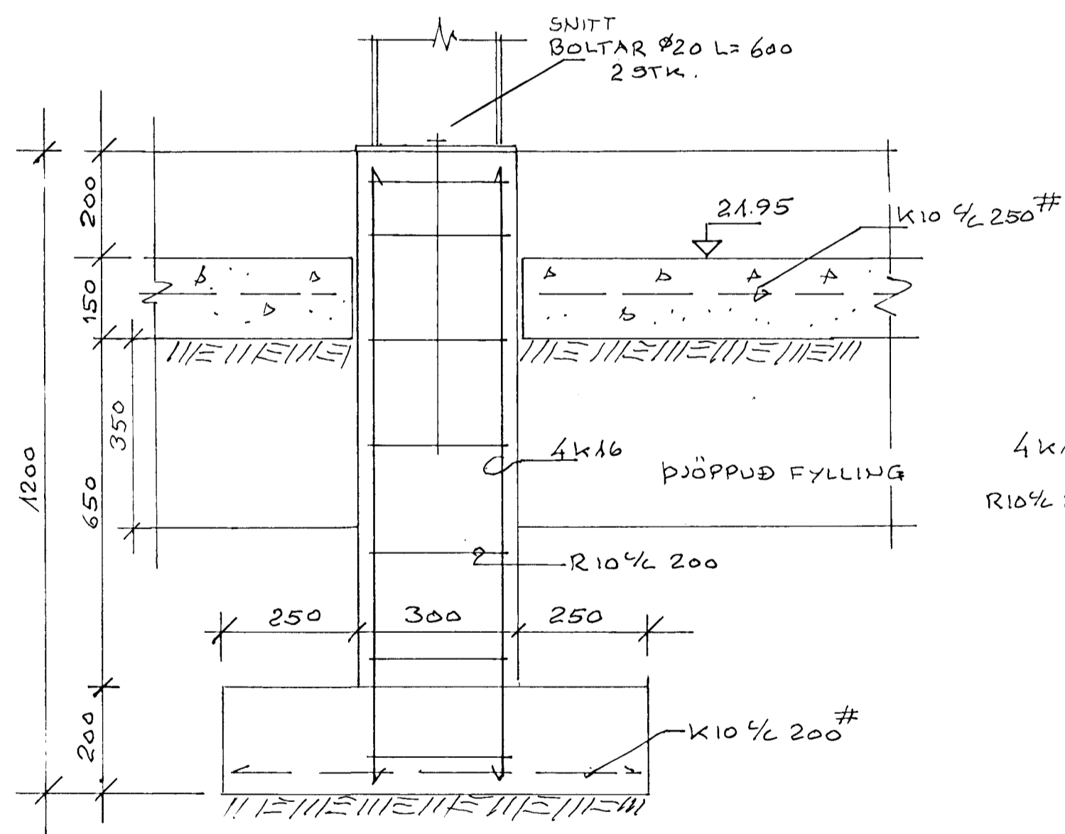
SNID B-B 1:10
