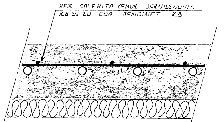
SÉRMÝND GÖLFHITA 1:5 Í GÖLFHITA SKAL NOTA 20 MM PEX 15 CM.
