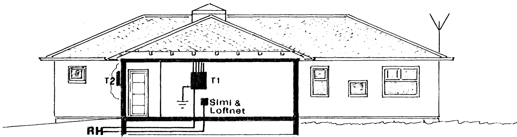
A - A 1:100
