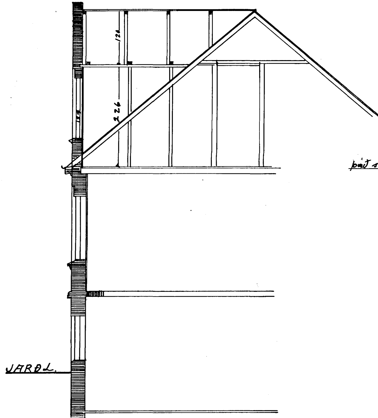
ÞVERSKURÐUR MALKV 1:50
