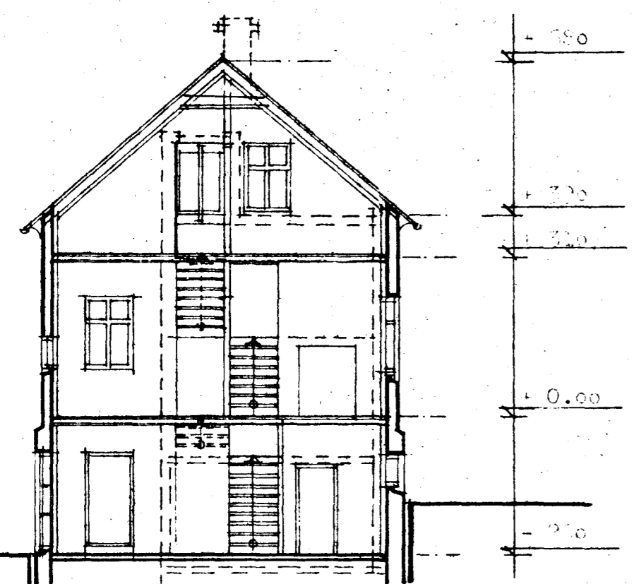
SNIDMYND AA
