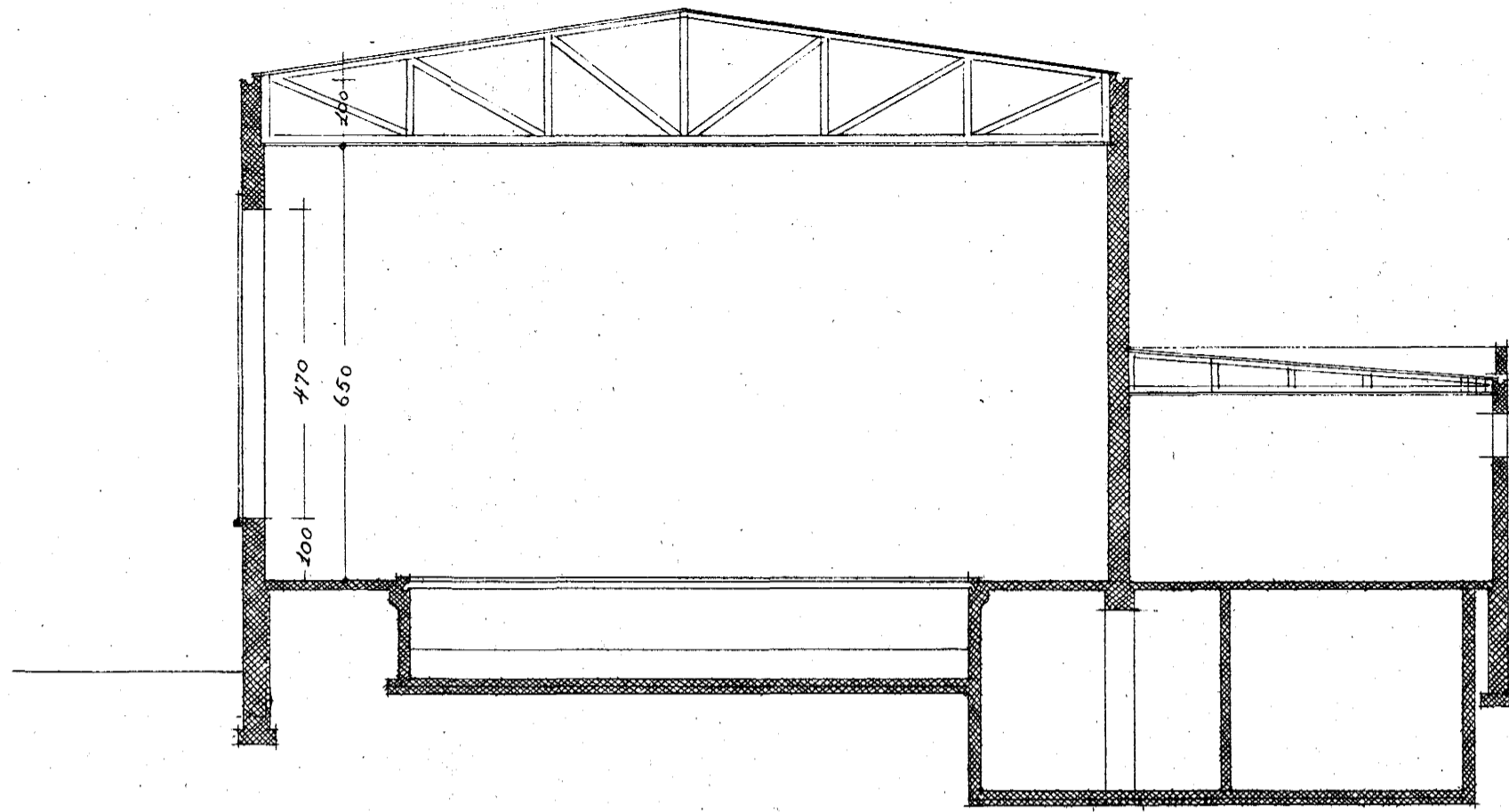
Þverskurður
