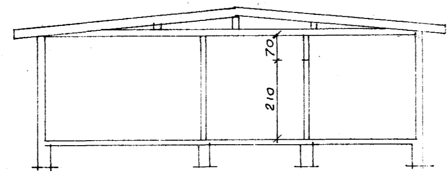
SKURÐUR
