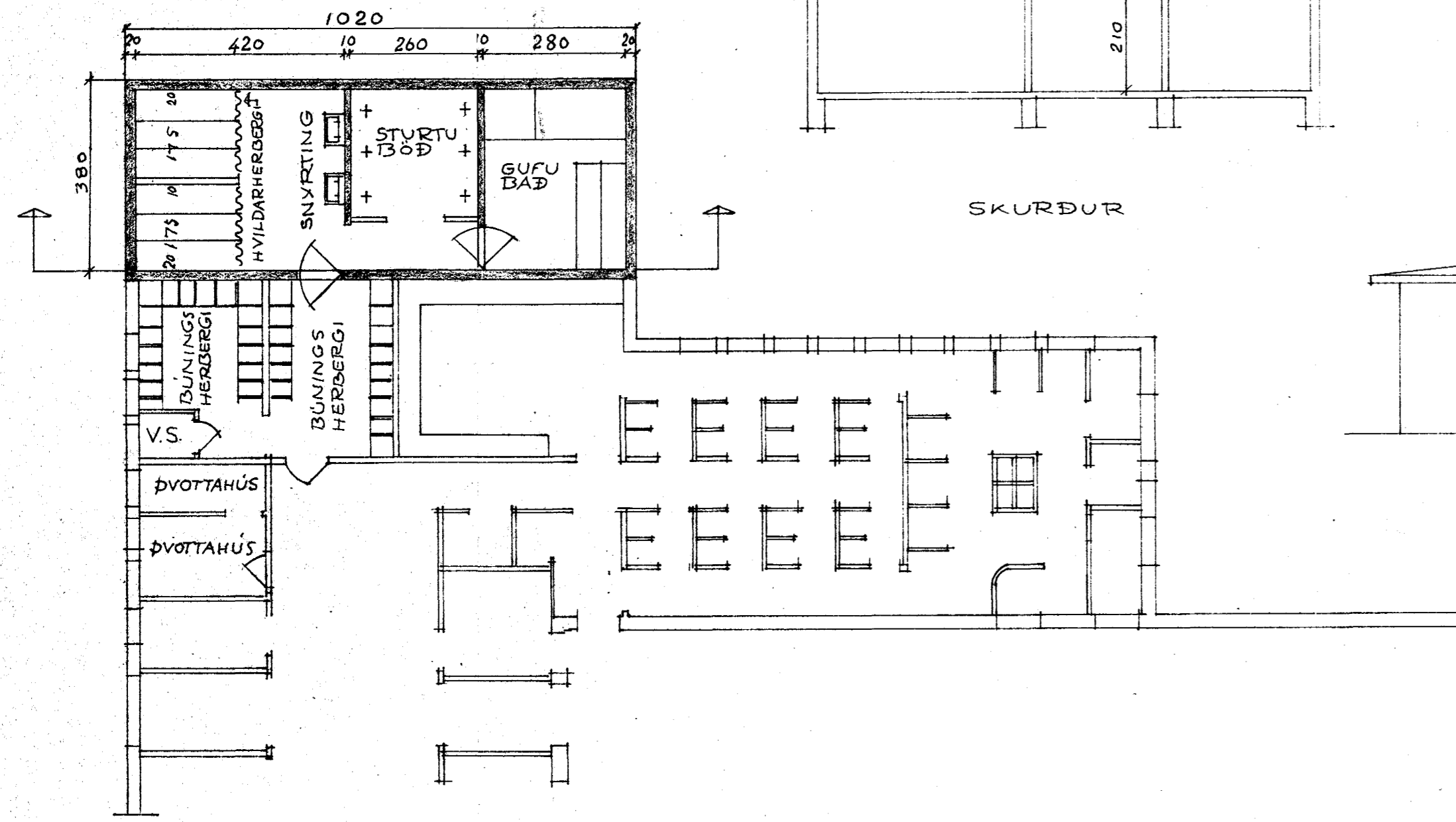
GRUNNMYND
