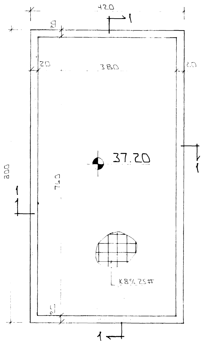
GRUNNM. UNDIRSTÖÐUR 1:50
