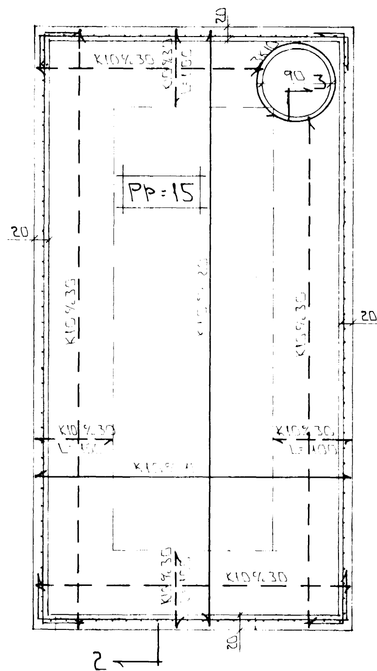
GRUNNMÝND 1:50
