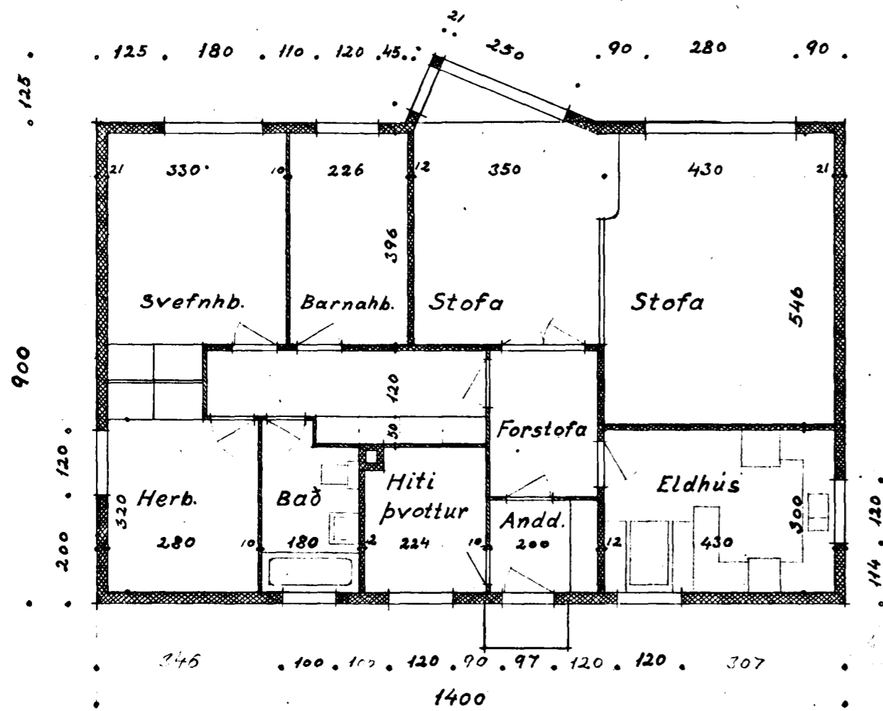
Grunnmynd.
