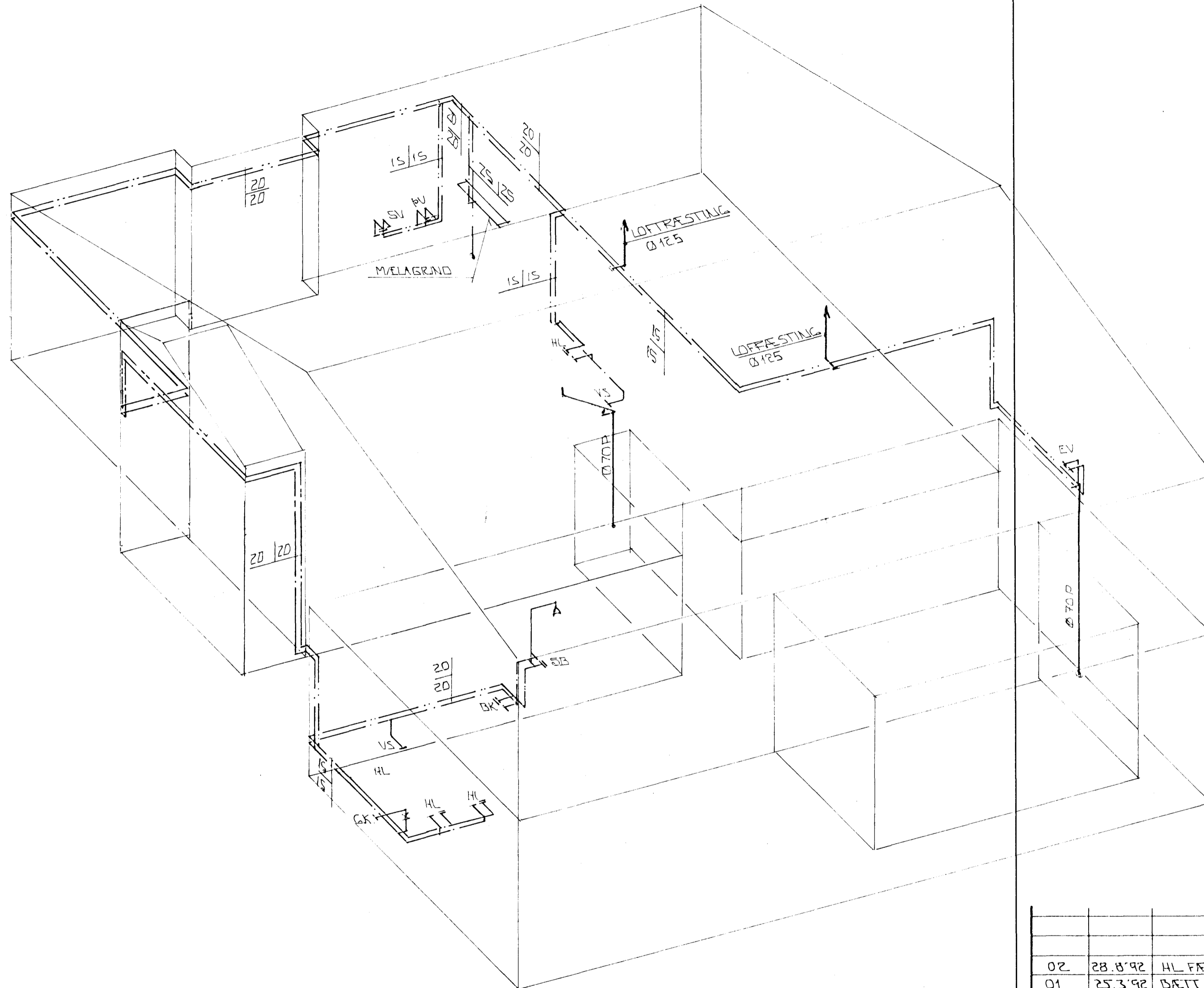
RÚMMYND VATNSLAGNA 1:50
