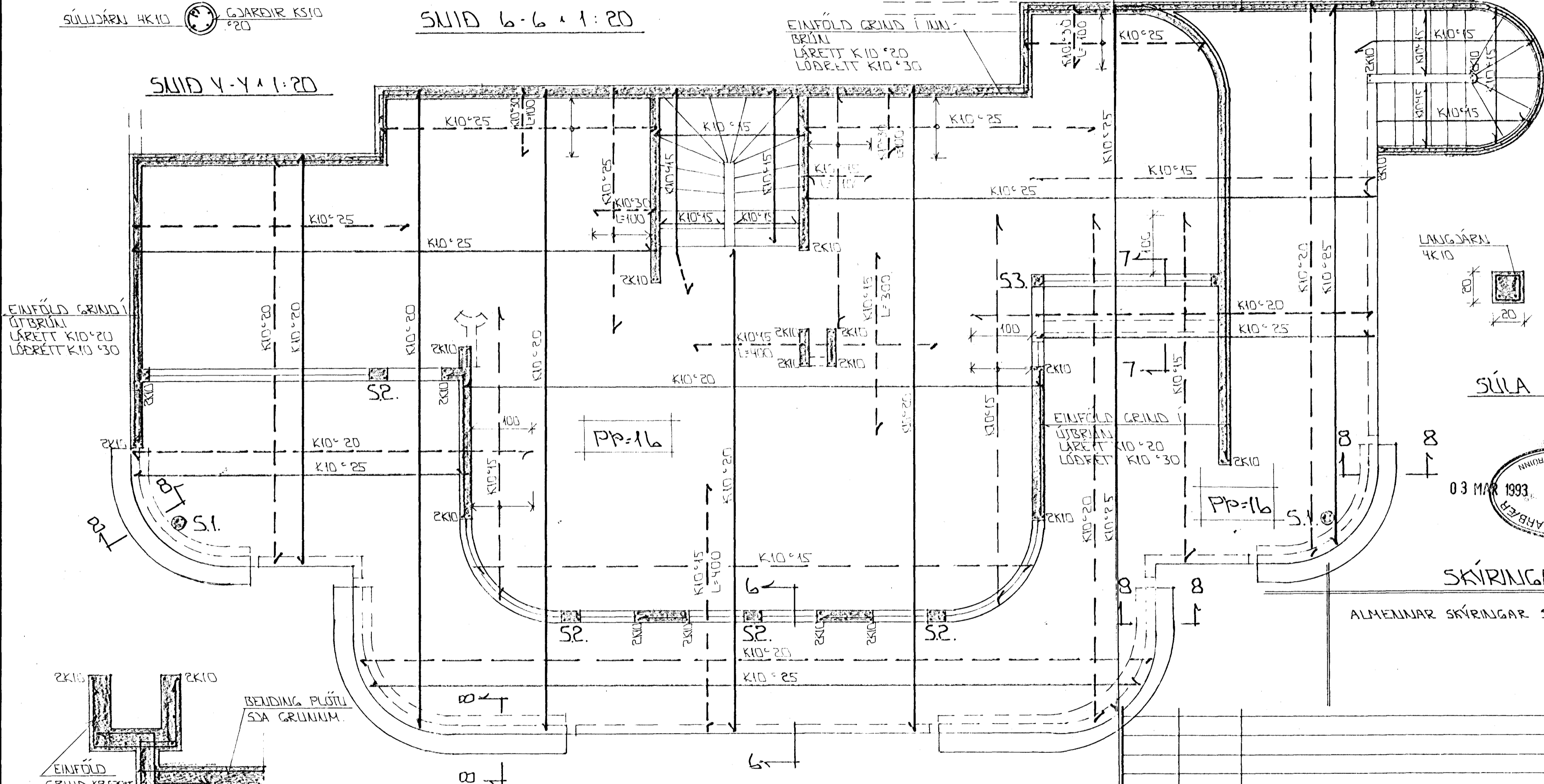
GRUNNMÝND 1:50
