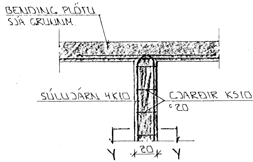
SÚLA S1 1:20
