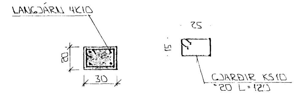
SÚLA S.2. 1:20
