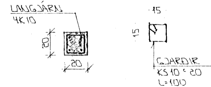
SÚLA S.3. 1:20
