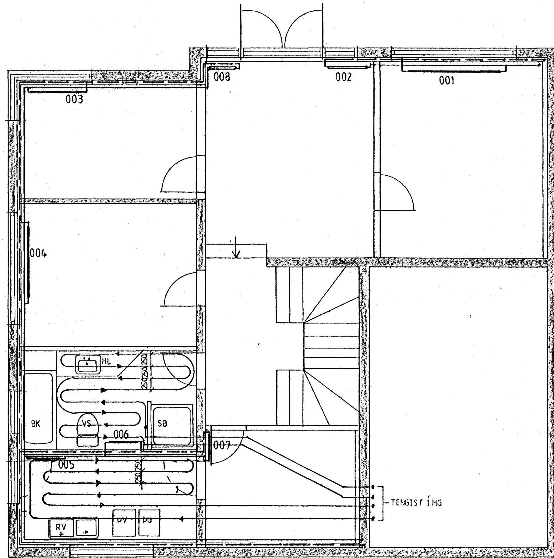
GRUNNMYND KJALLARA. OFNAR. M=1:50
