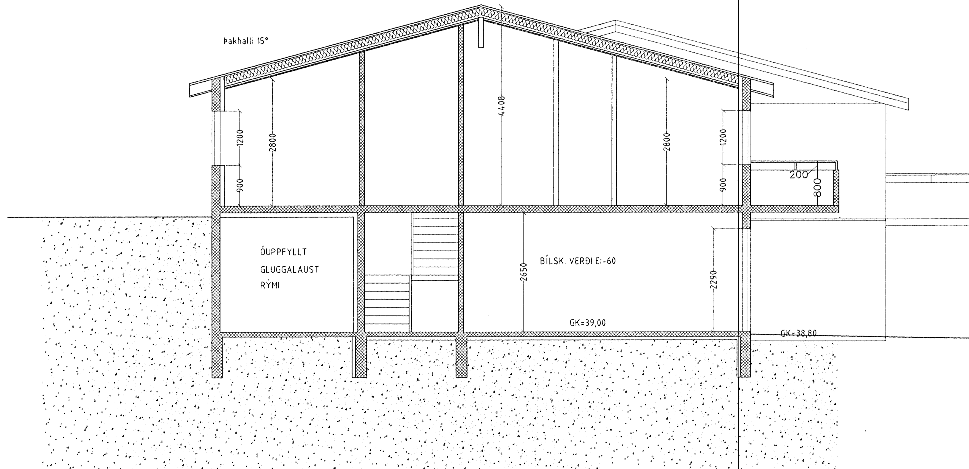
SNID A-A
