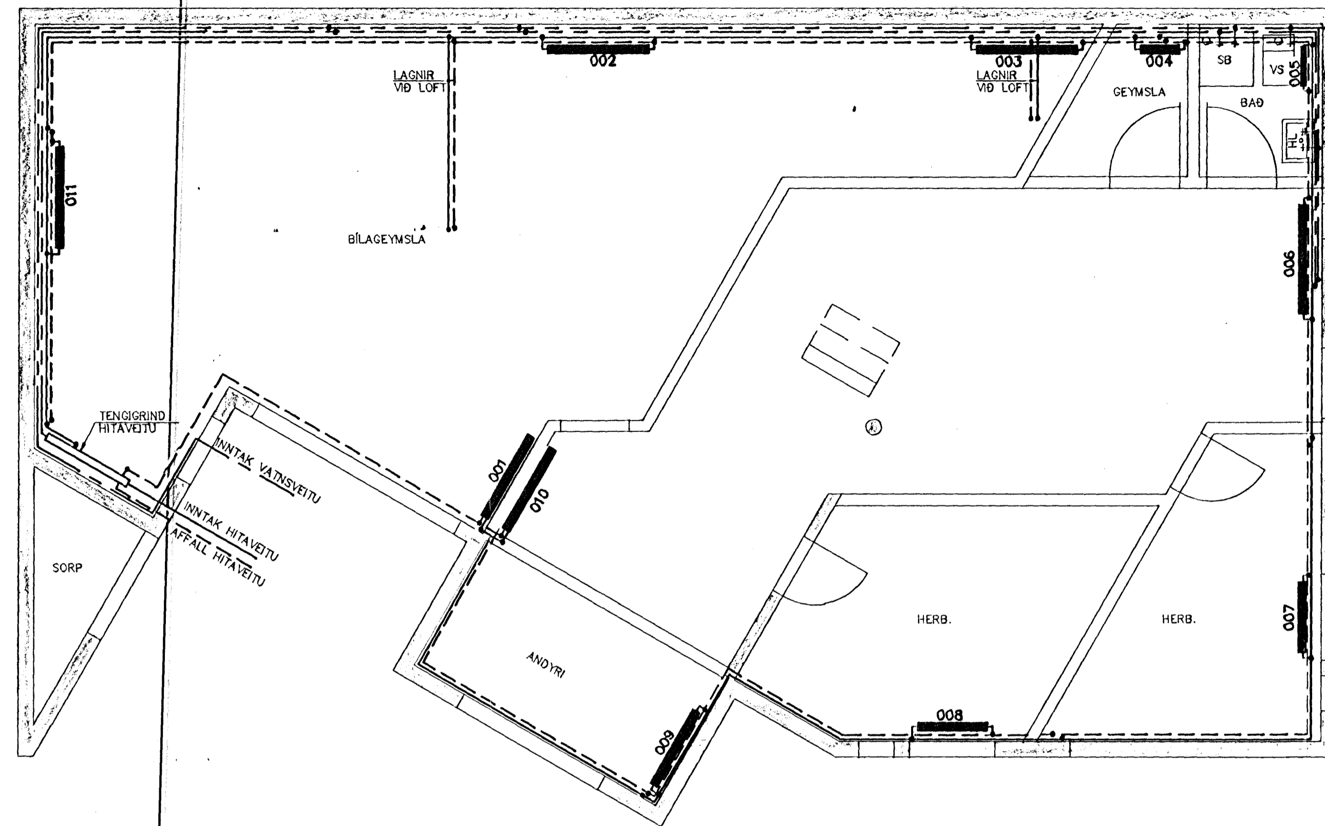
GRUNNMYND JARÐHÆÐAR 1:50
