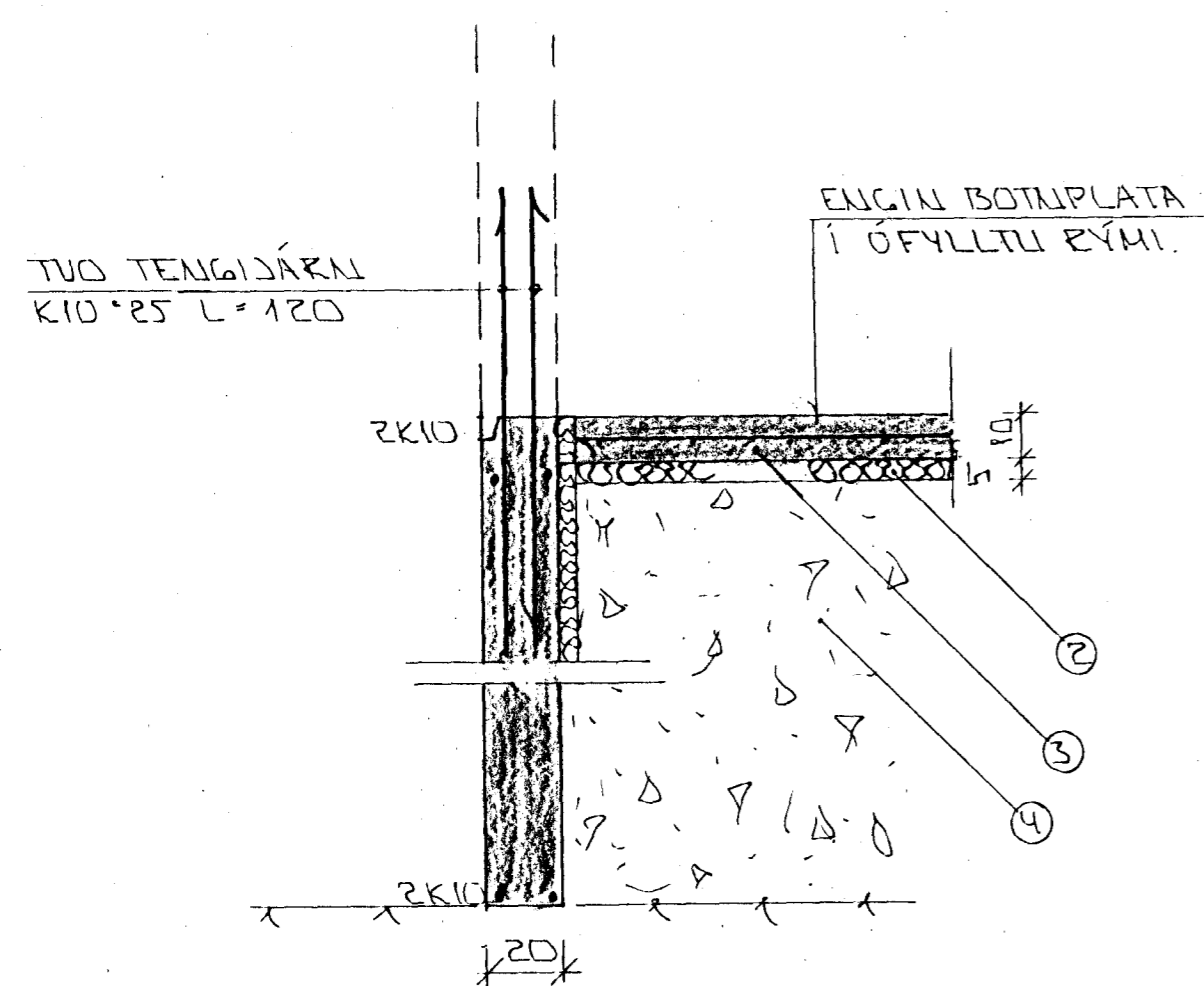
SNID 2 1:20
