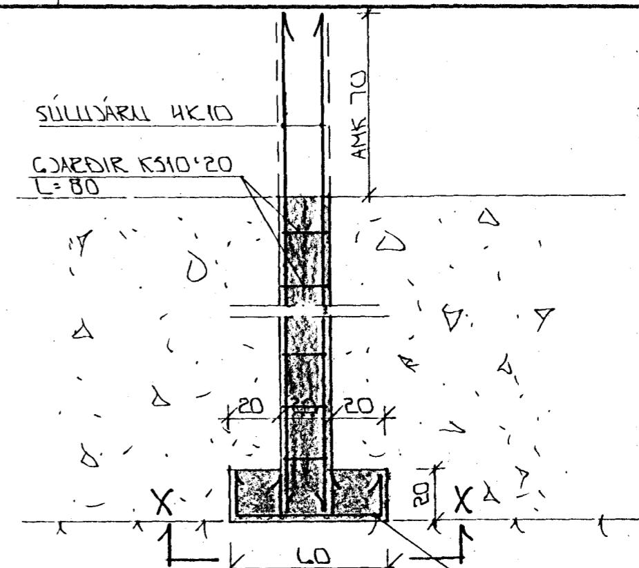
SÚLA S1 1:20
