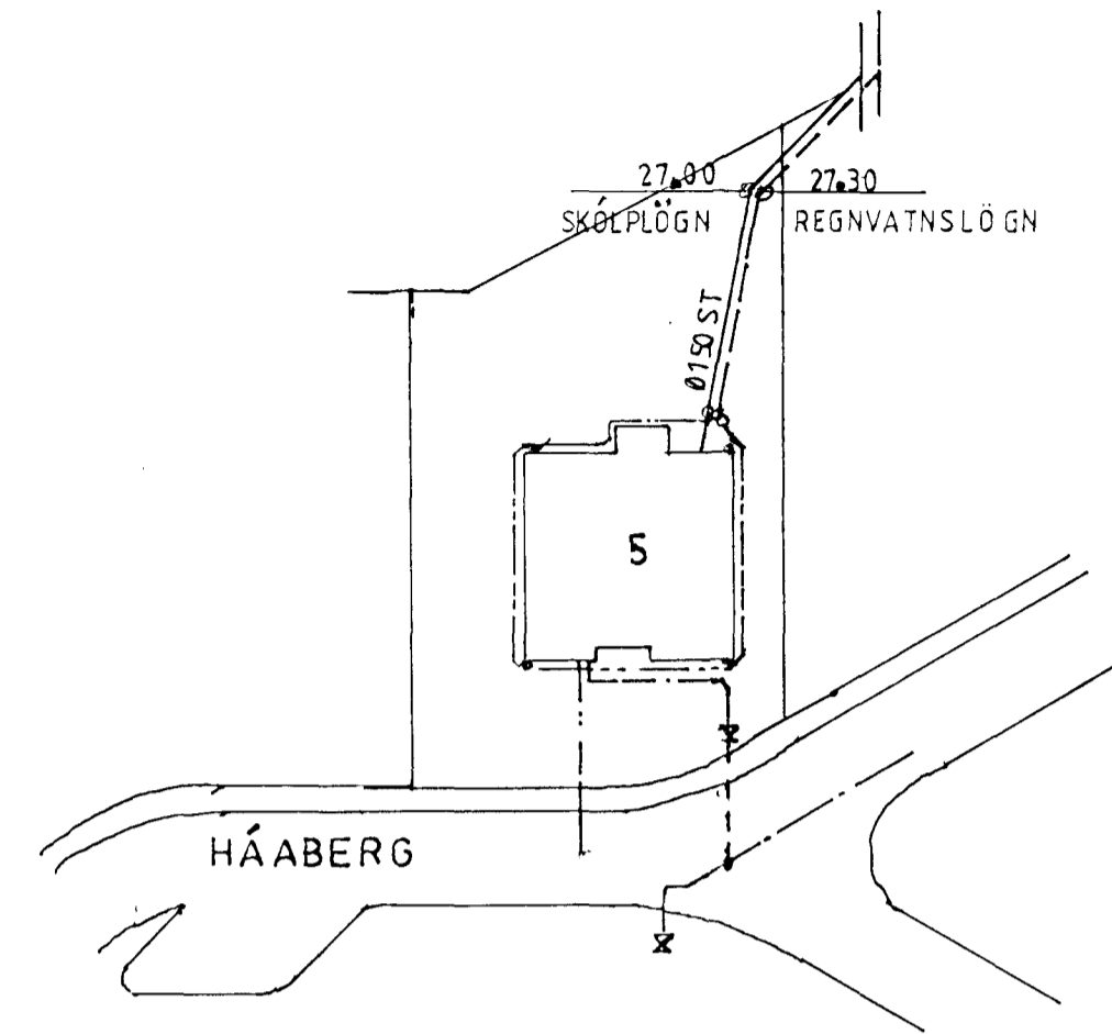
AFSTÖÐUMYND M:1:500
