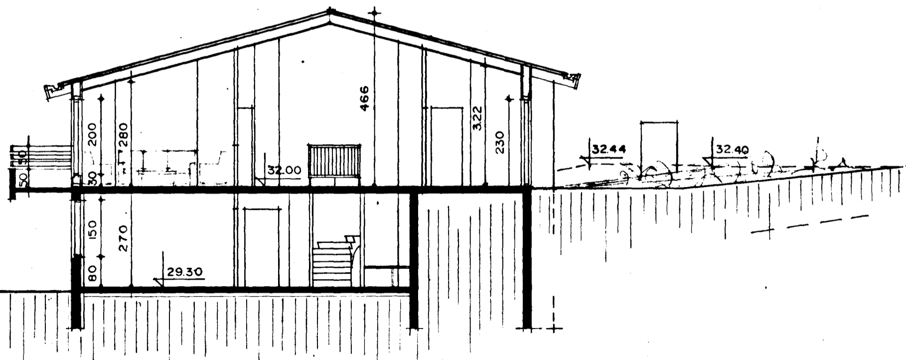
SNIÐ A-A M.1:100
