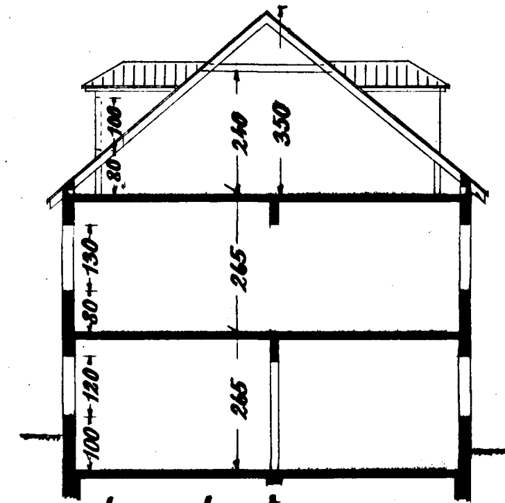
Þverskurður
