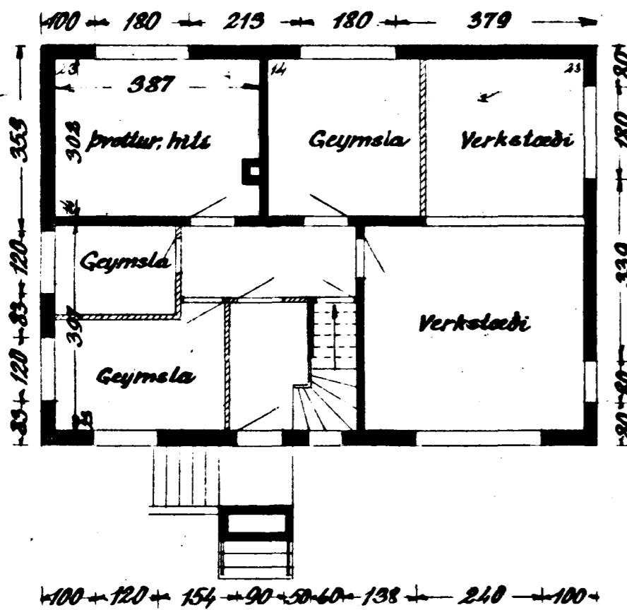
Kjallari
