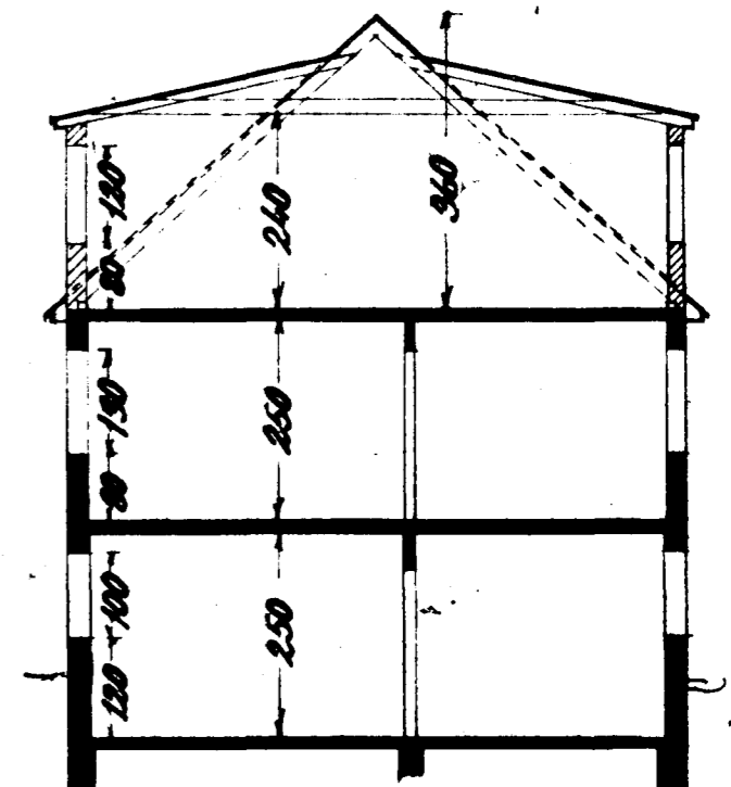
Þverskurður
