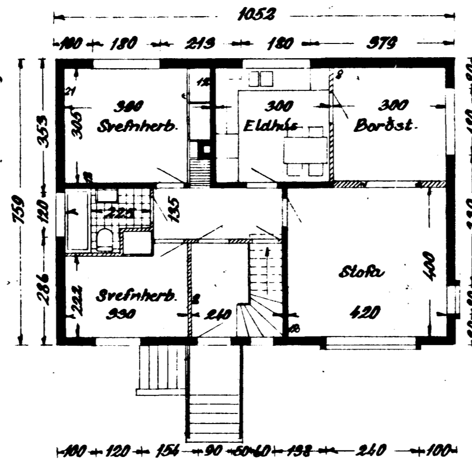
Hæð
