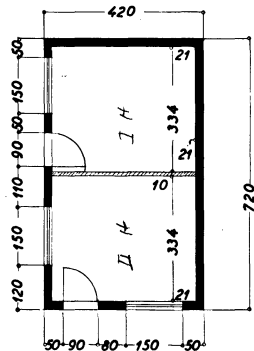
Grunnmynd
