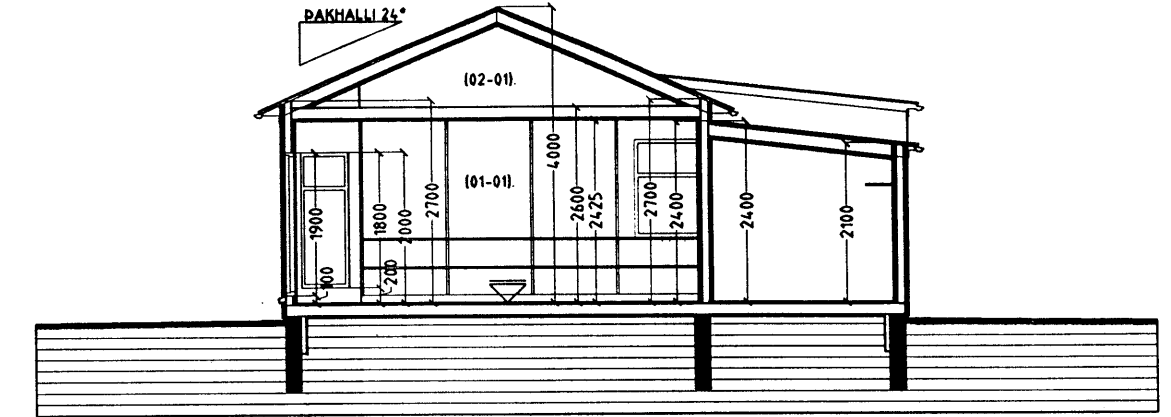
SNID A-A MKV. 1:100
