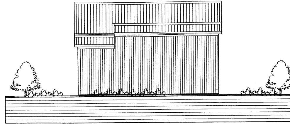
ÚTLIT NORÐVESTUR MKV. 1:100
