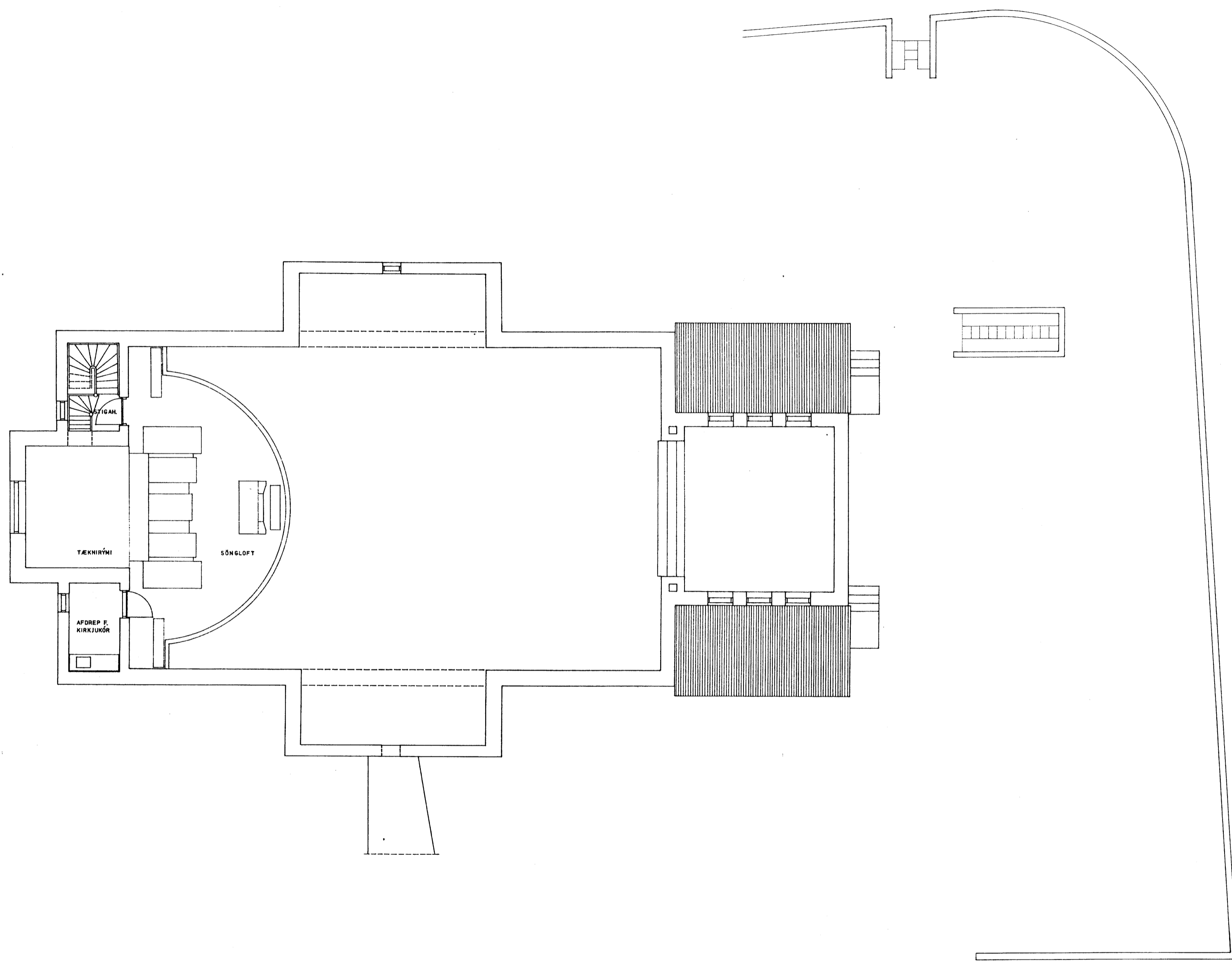
GRUNNMYND SÖNGLOFTS
