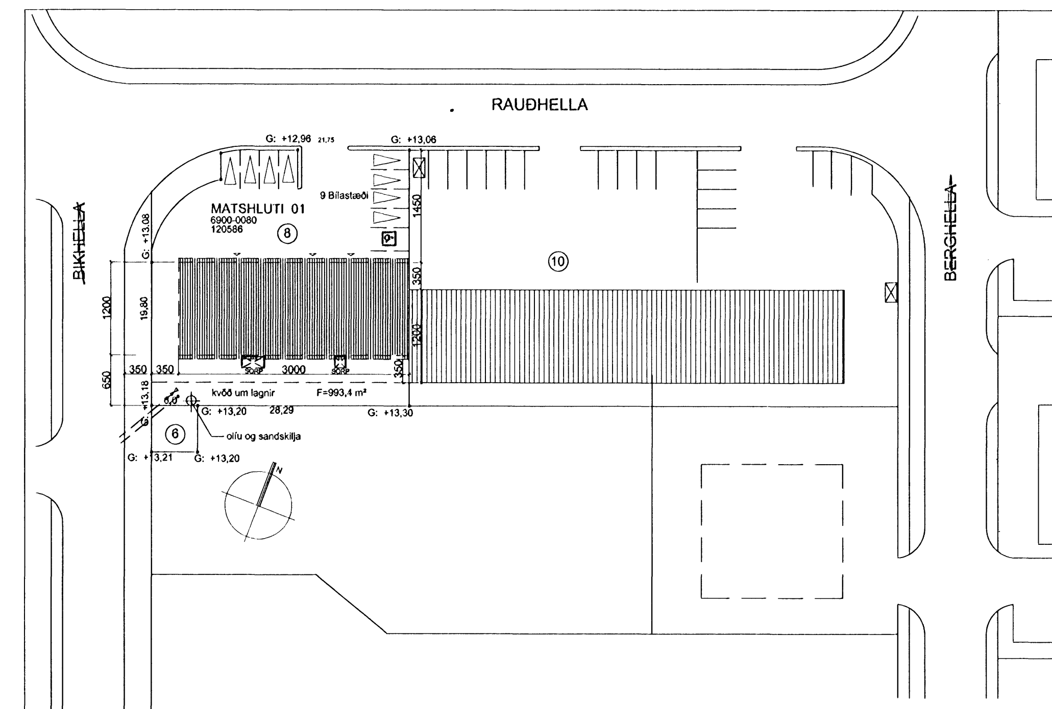
AFSTÖÐUMYND 1:500
