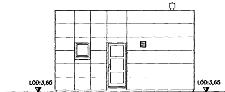
VESTURHLID MKV. 1
