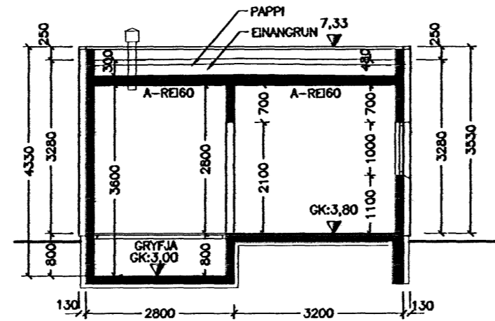
1 SNID MKV. 1
