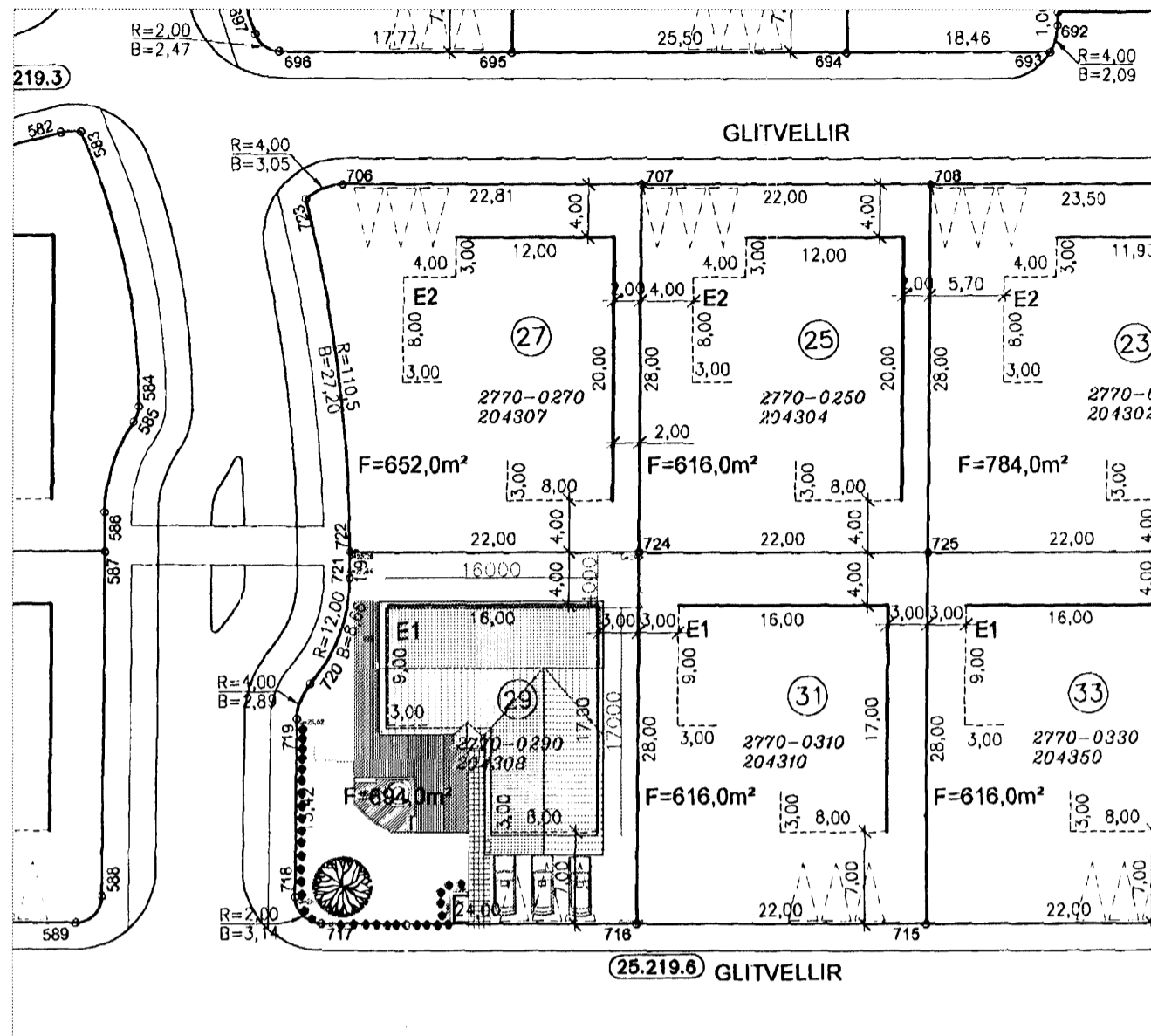
Afstöðumynd 1.500
