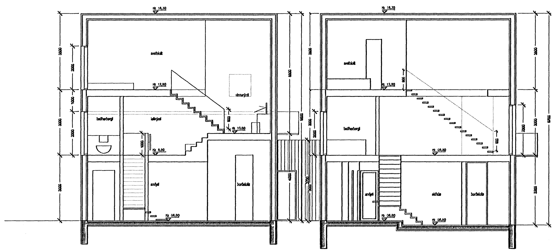
sneiðing a 1:100
