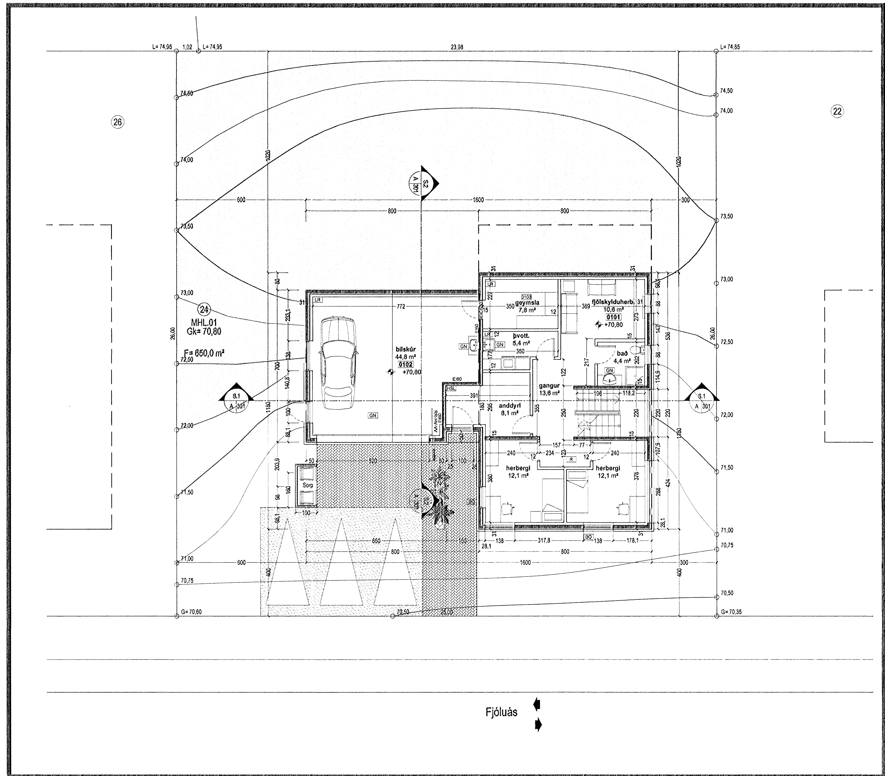
Grunnmynd 1 hæð 1:100
