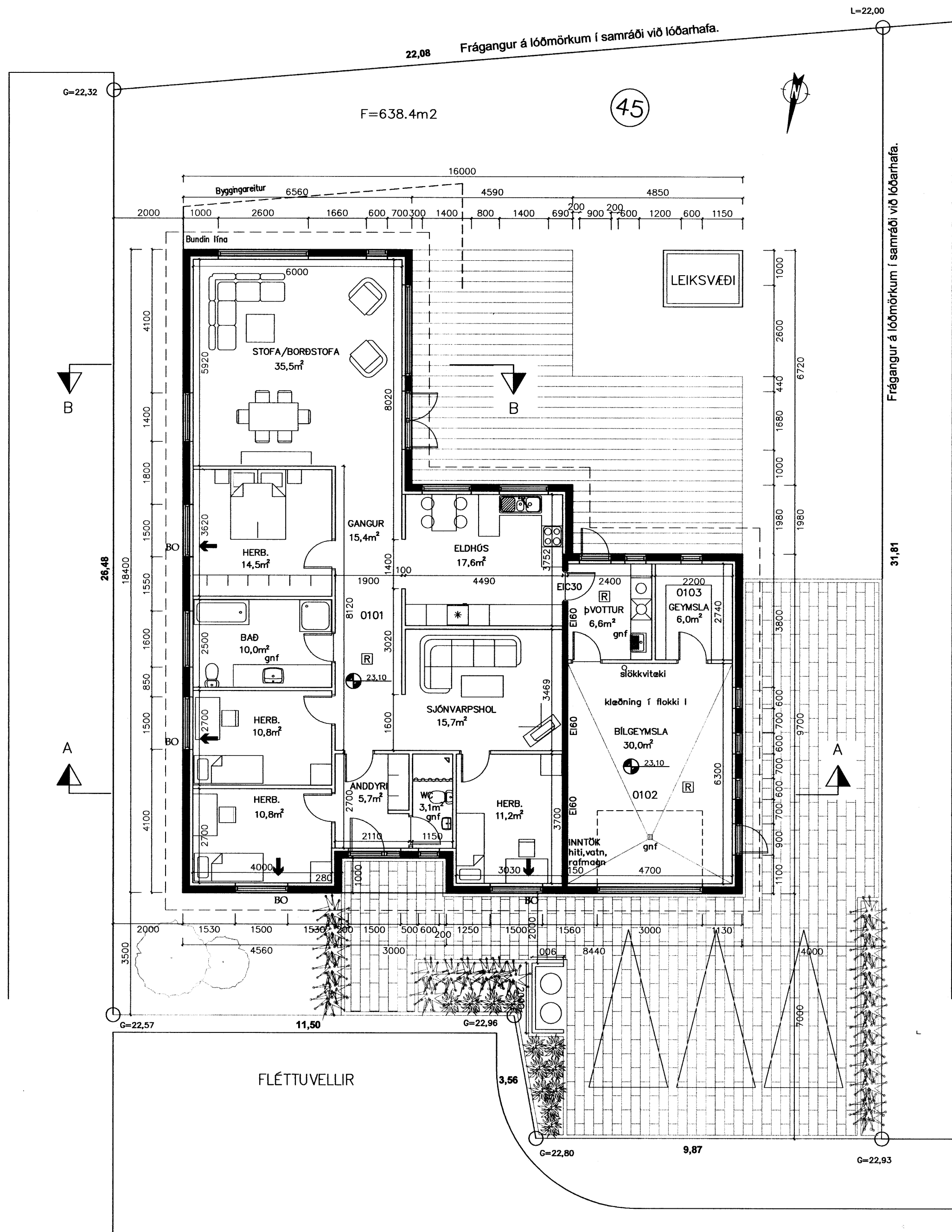
GRUNNMYND 1:100
