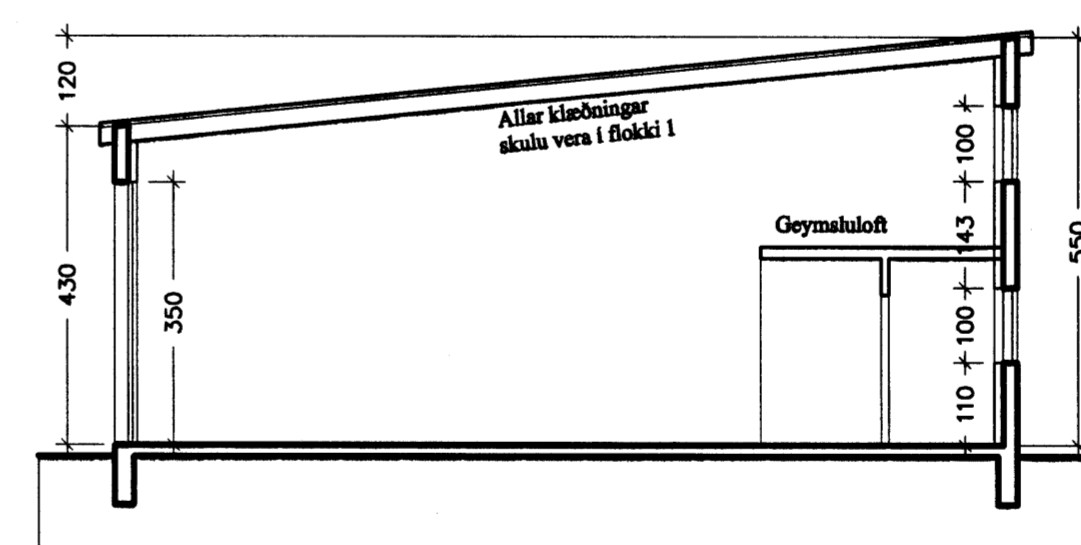
SNEIÐING 1:100
