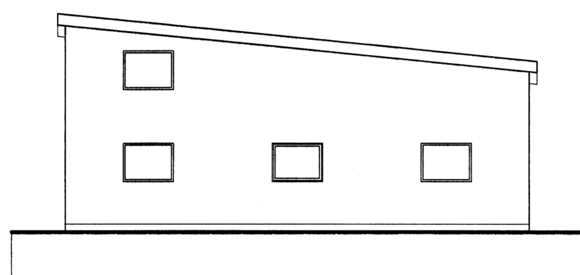
ÚTLIT AUSTUR 1:100
