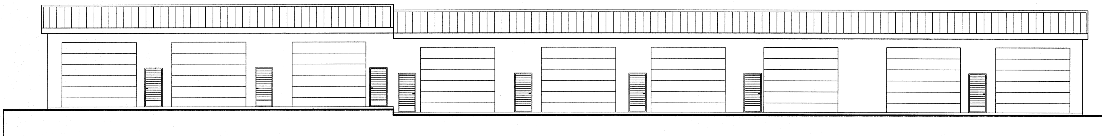
ÚTLIT SUÐUR 1:100
