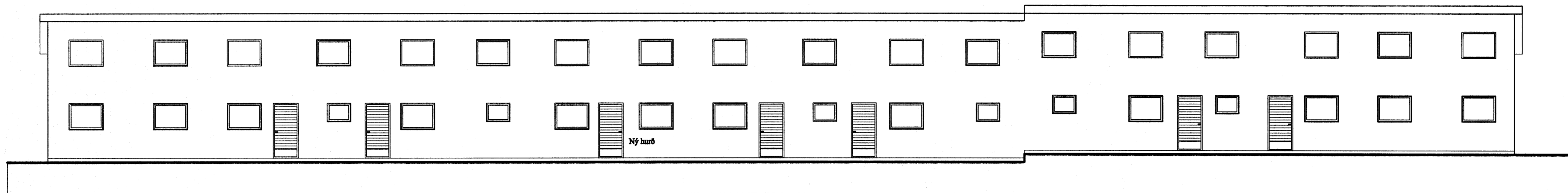
ÚTLIT NORÐUR 1:100
