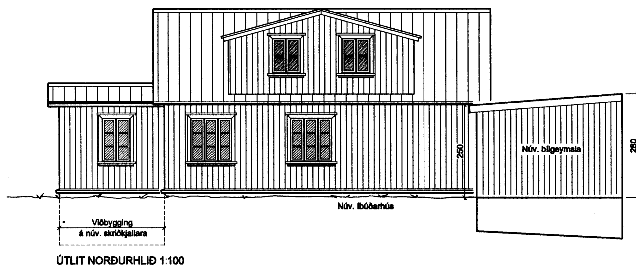
ÚTLIT NORÐURHLÍÐ 1:100
