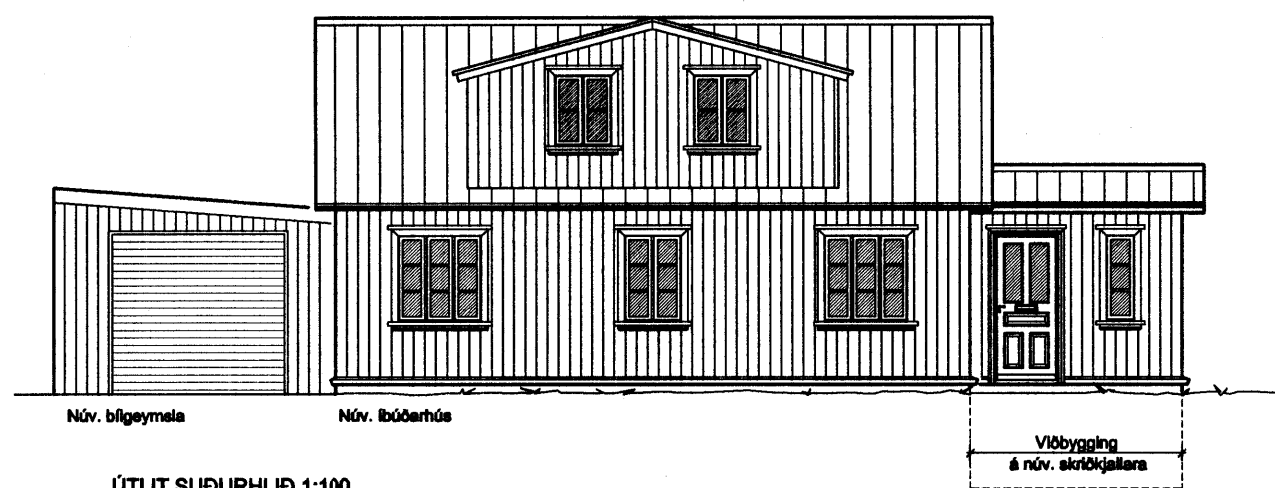
ÚTLIT SUÐURHLÍÐ 1:100
