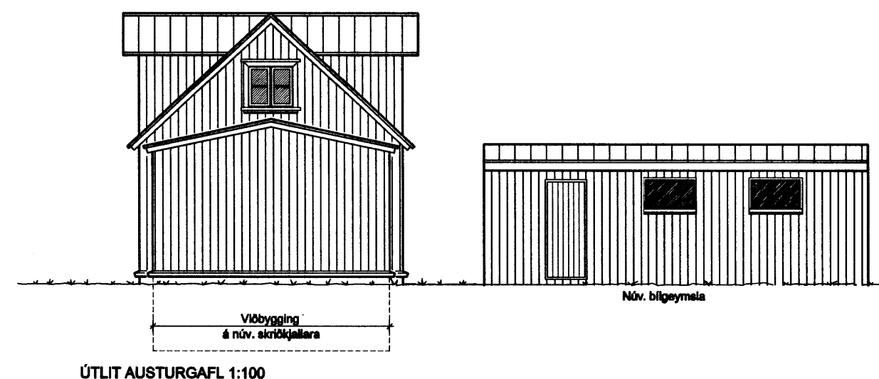
ÚTLIT AUSTURGAFL 1:100
