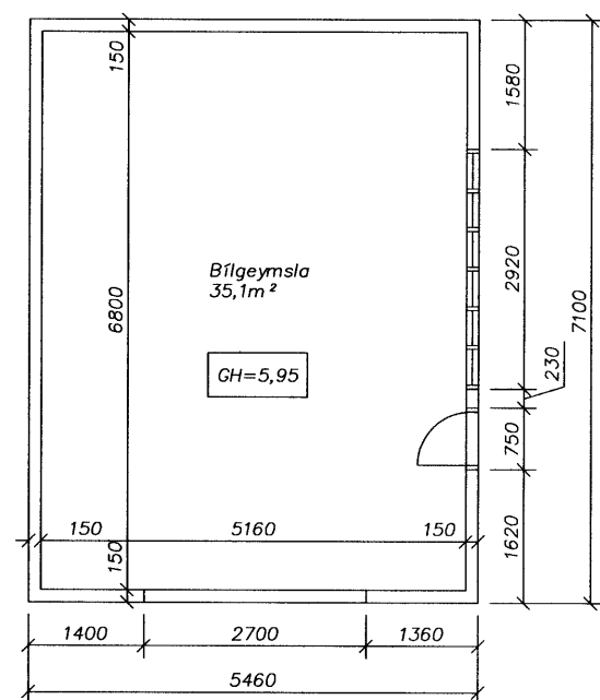
Grunnmynd Mælikvarði 1:100
