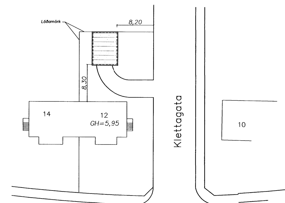
Afstaða Mælikvarði 1:500
