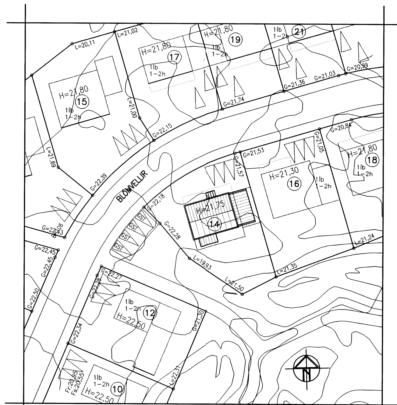
AFSTÖÐUMYND 1:500
