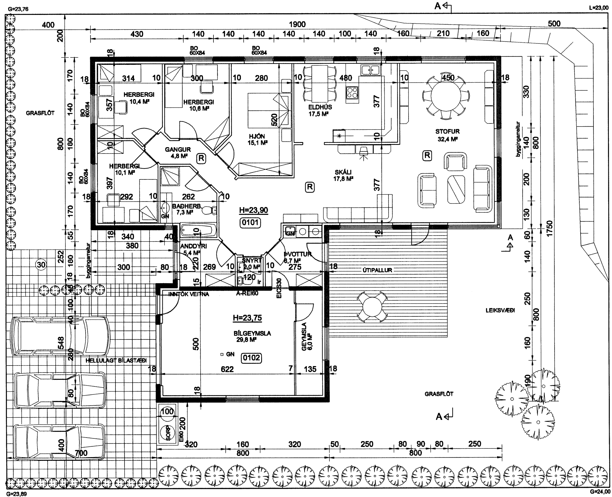
GRUNNMYND MKV. 1:100
