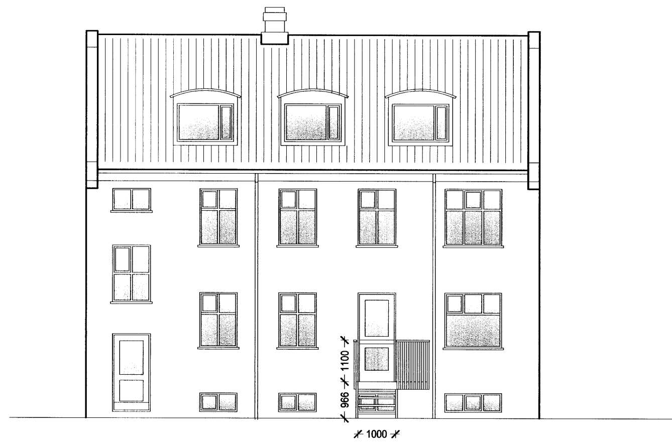
Útlit, suður mkv. 1:100
