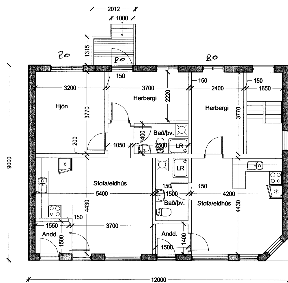
Grunnmynd 1. hæðar mkv. 1:100
