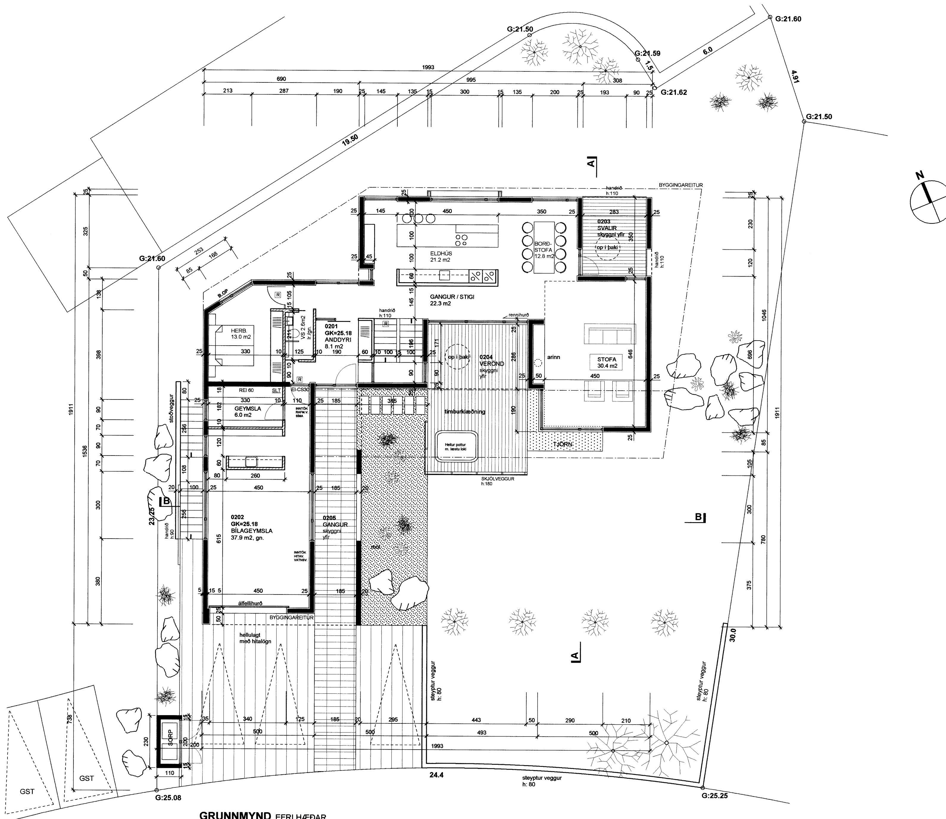
GRUNNMYND EFRÍ HÆÐAR
