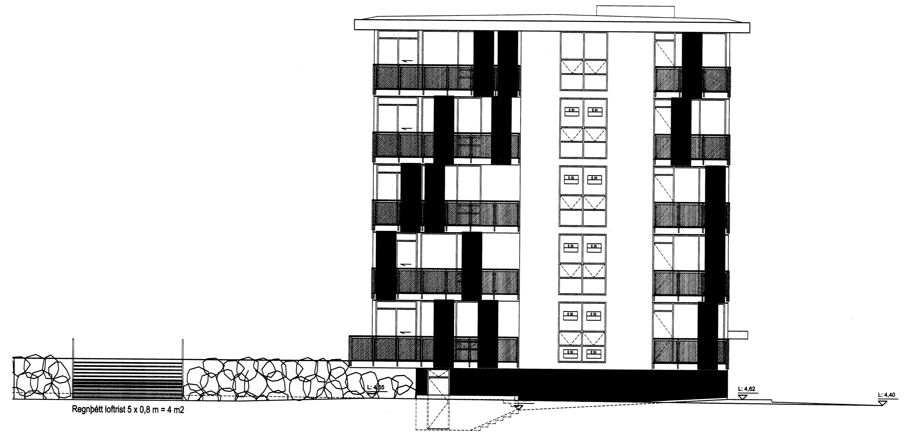
17-SUÐVESTURHLIÐ í mkv. 1:100
