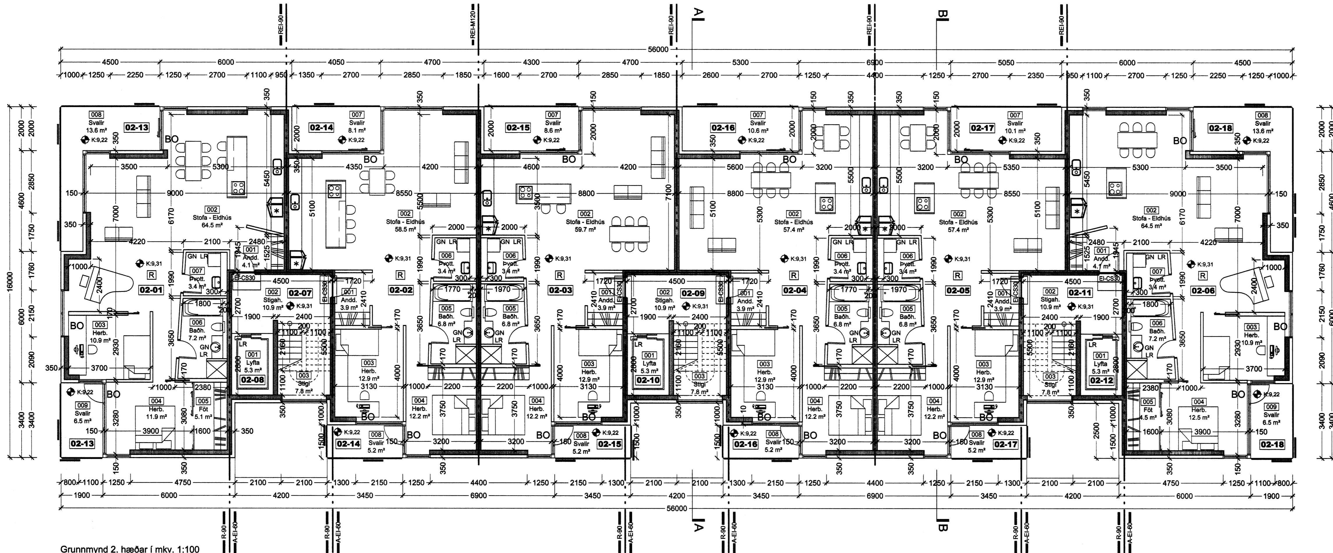
Grunnmynd 2. hæðar í mkv. 1:1000
