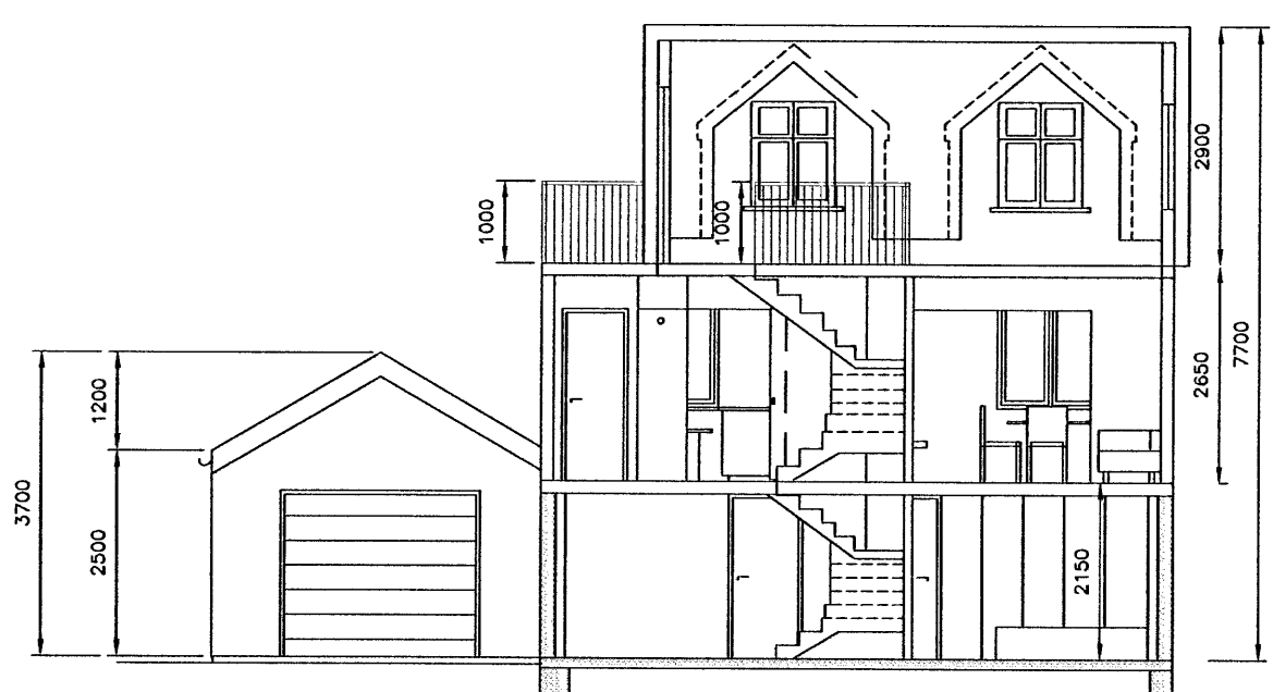
SNID A-A 1:100
