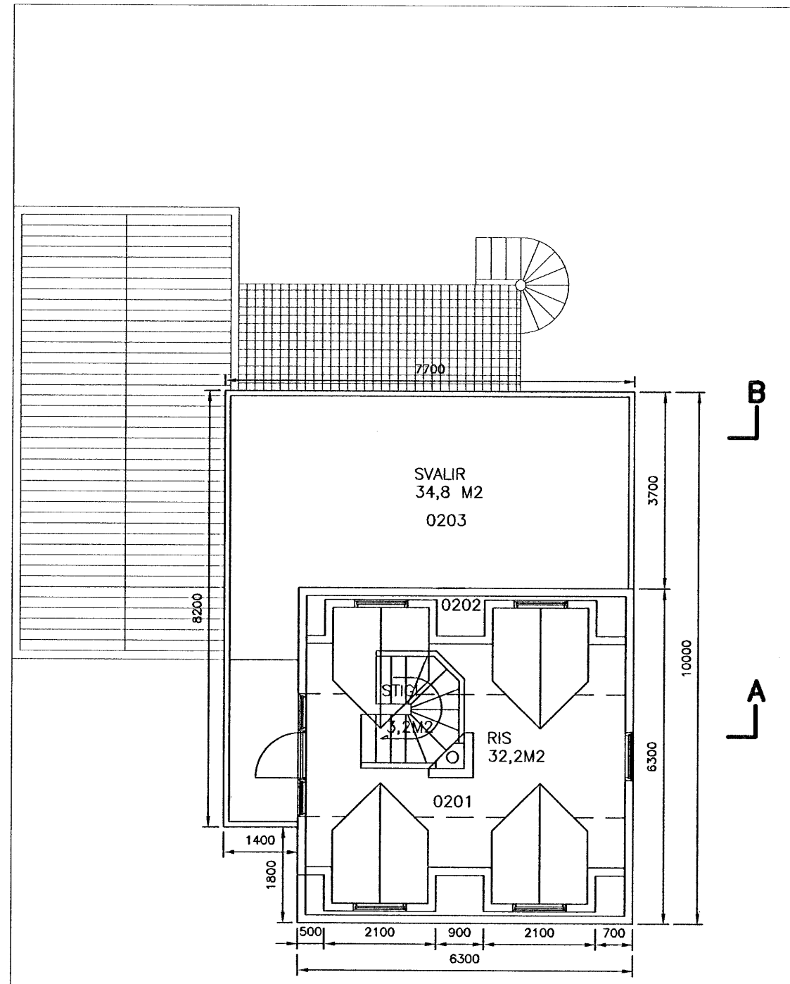
GRUNNMYND. RIS 1:100
