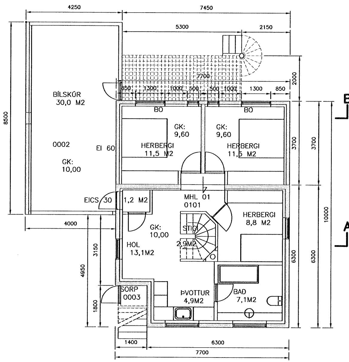
GRUNNMYND. KJALLARI 1:100
