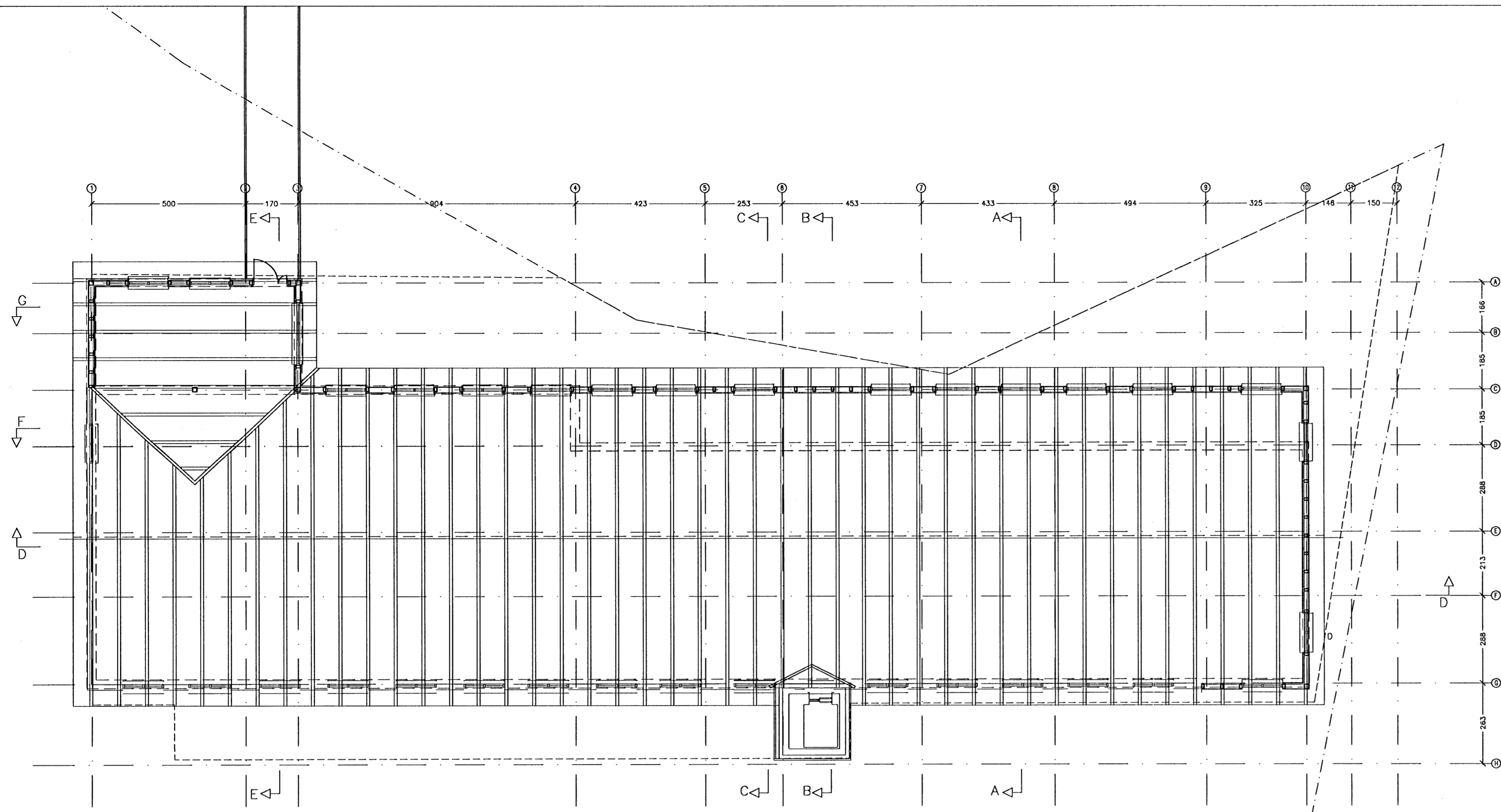
Grunnmynd þak sperrur. mskv. 1:100.
