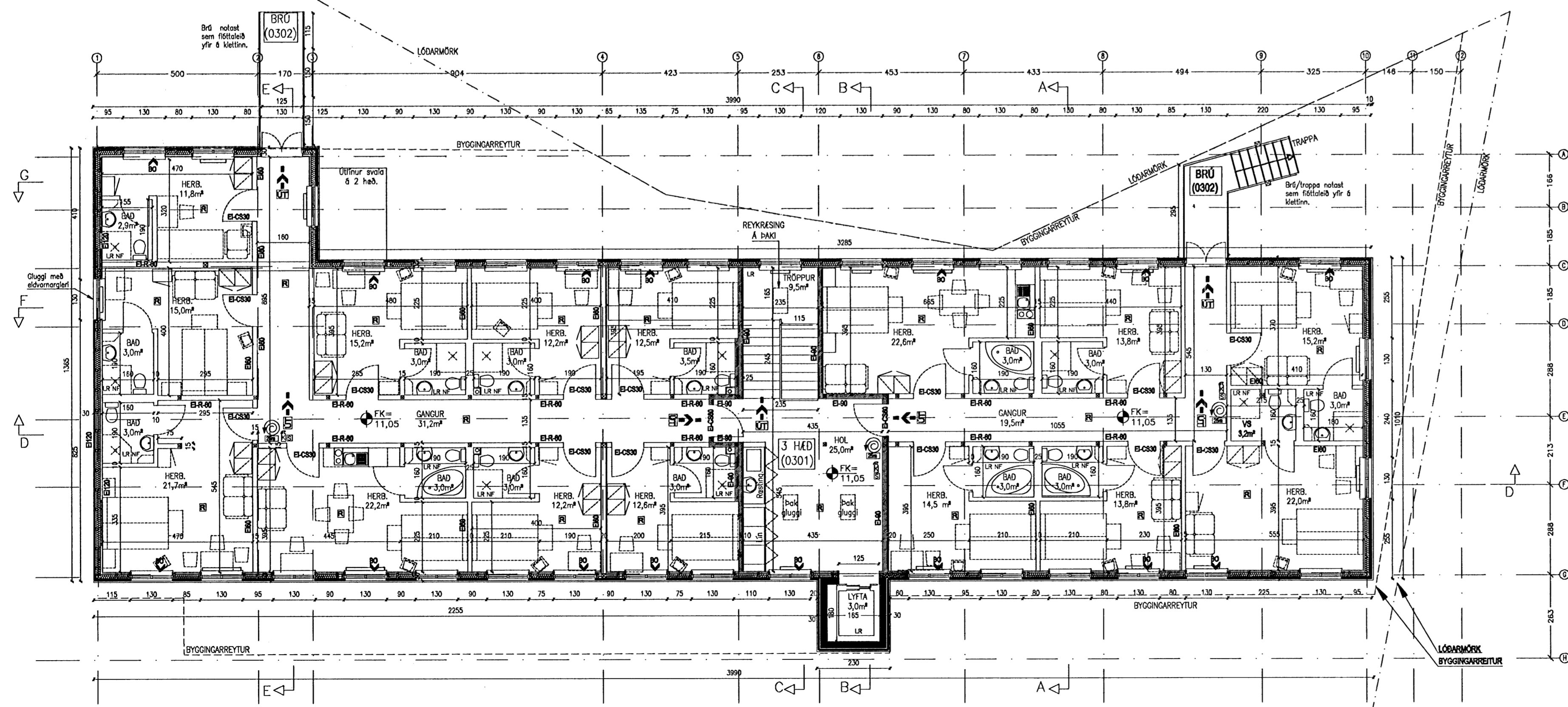
Grunnmynd 3. hæð. mskv. 1:100.
