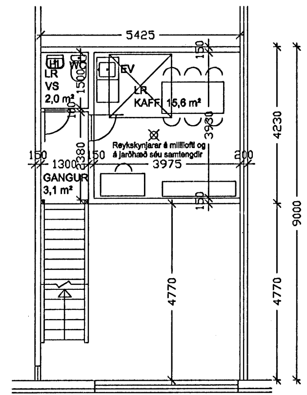
GRUNNMYND MILLILOFT MKV. 1:100
