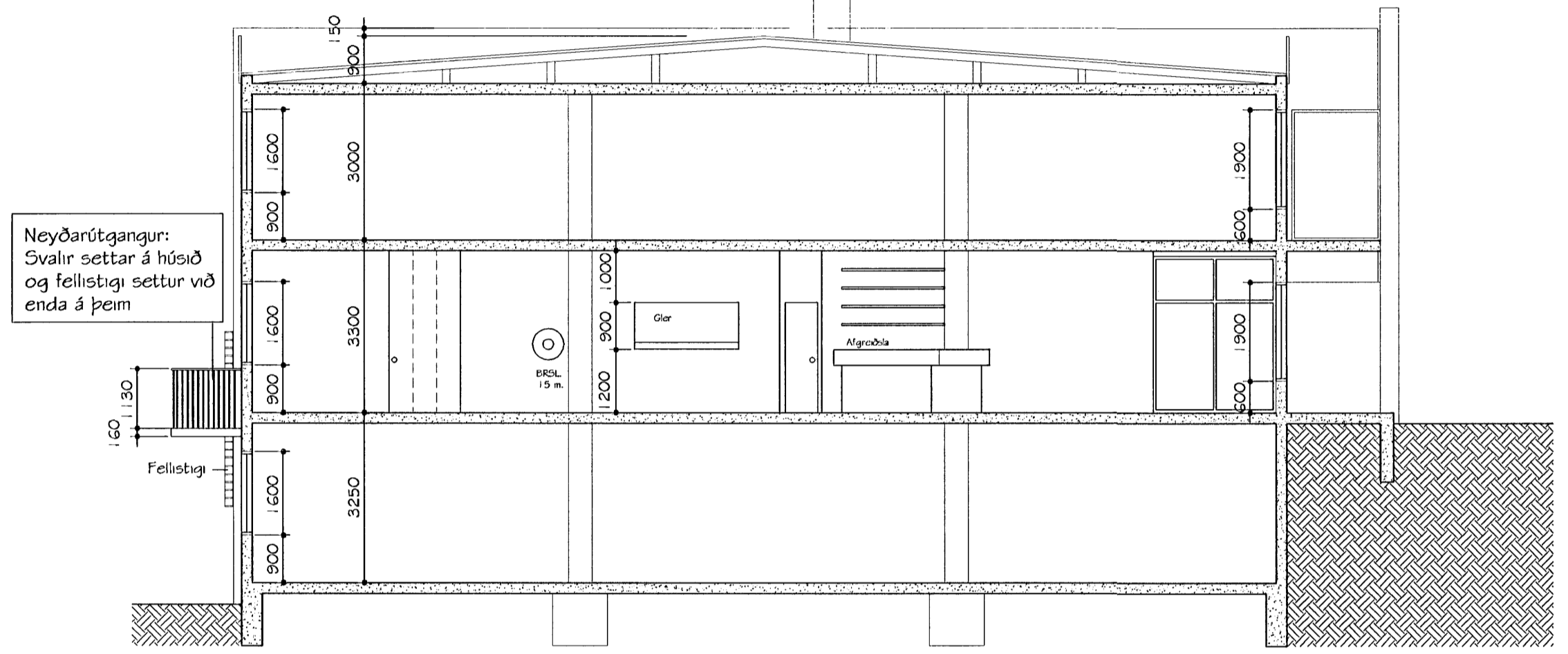
SNEIÐING A-A
