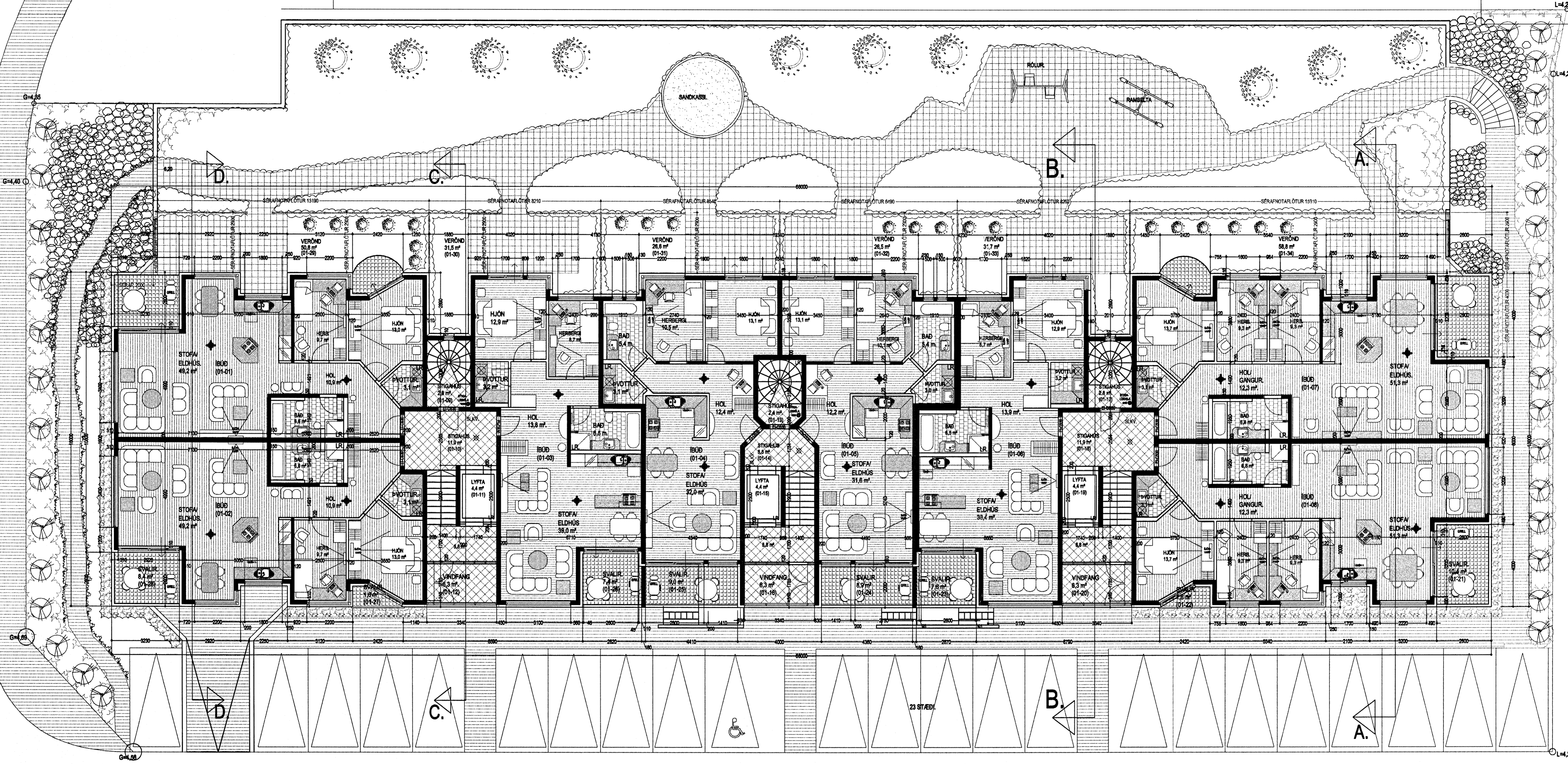
GRUNNMYND 1. HÆÐ. MKV. 1:100.
