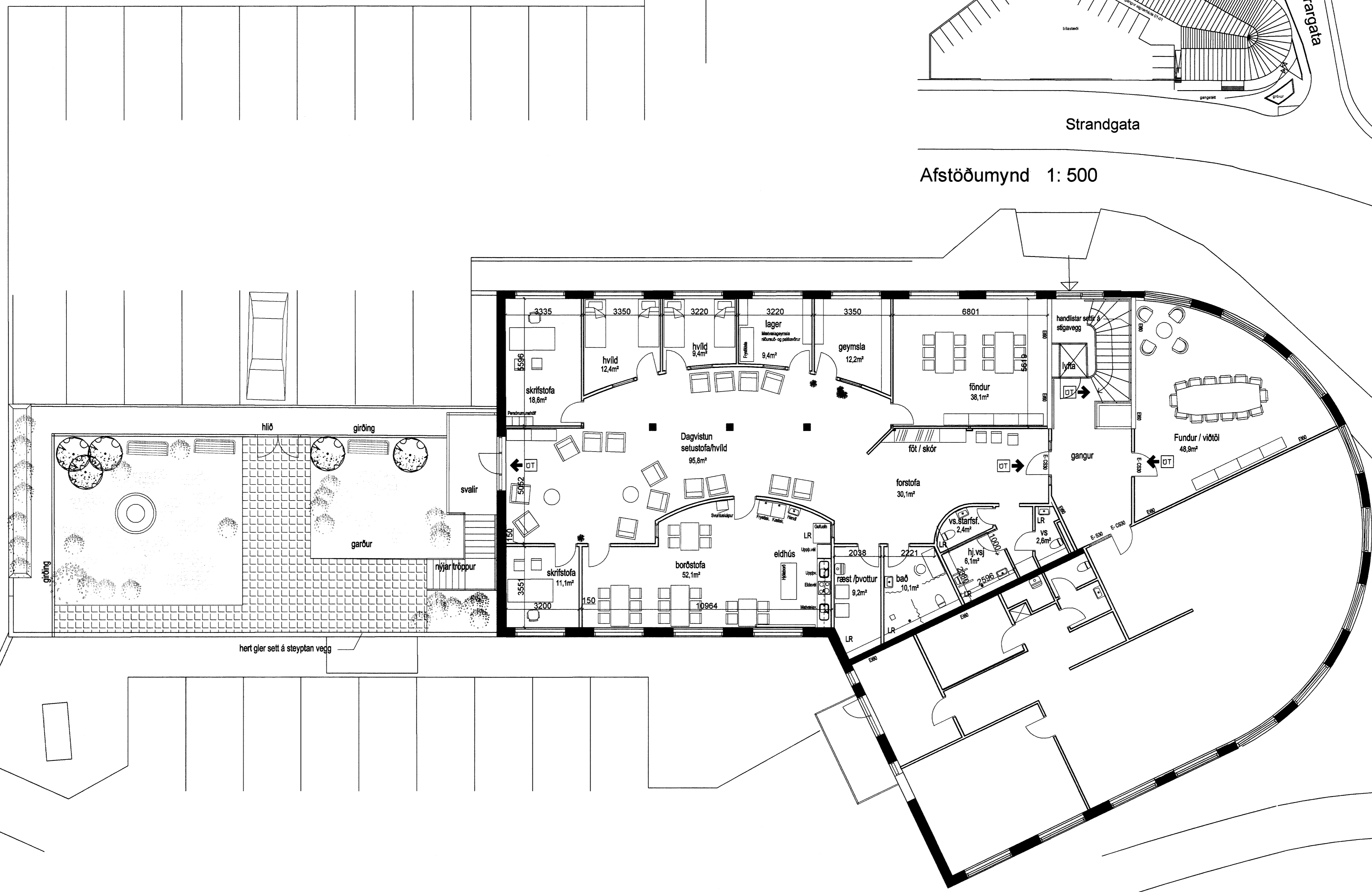
Grunnmynd 3. hæðar 1:100
