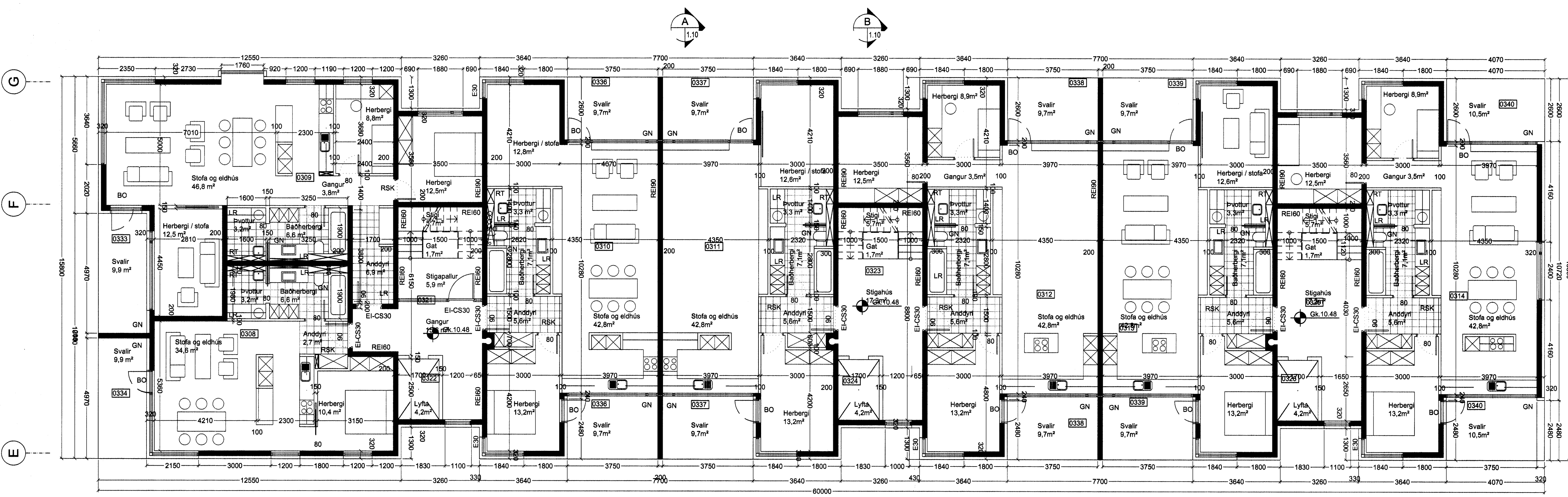
Grunnmynd 3. hæð, Norðurbakki 3.
