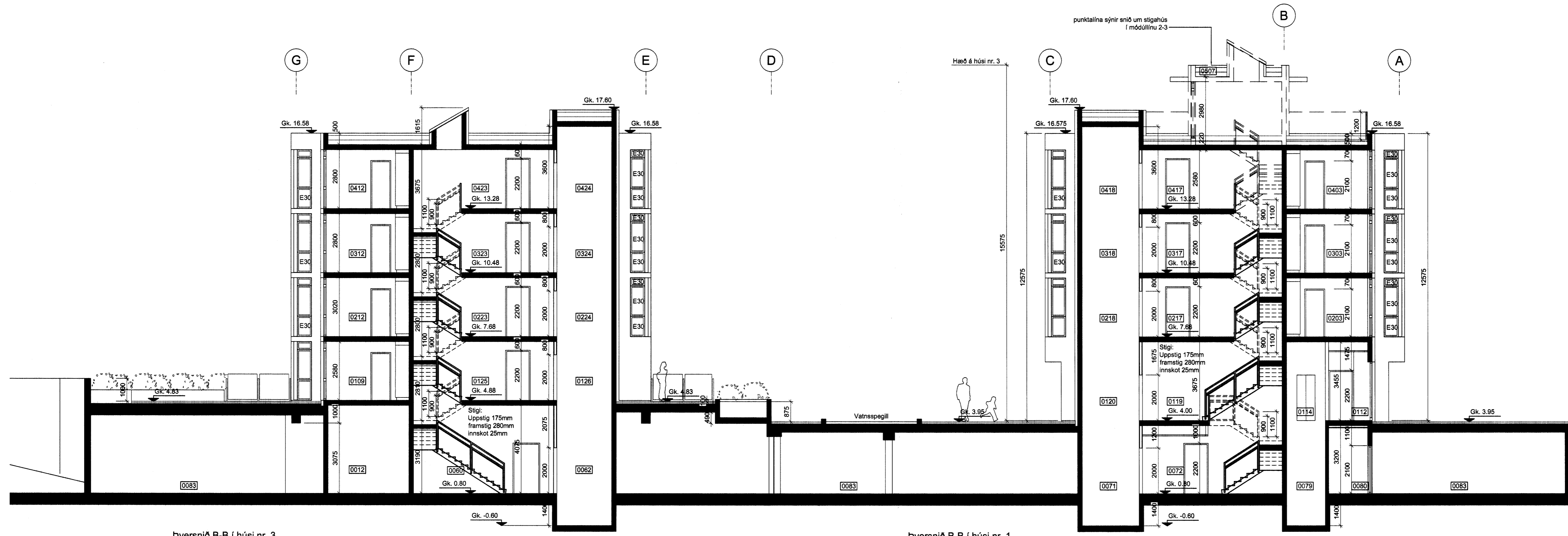
Þversnið B-B í húsi nr. 3
