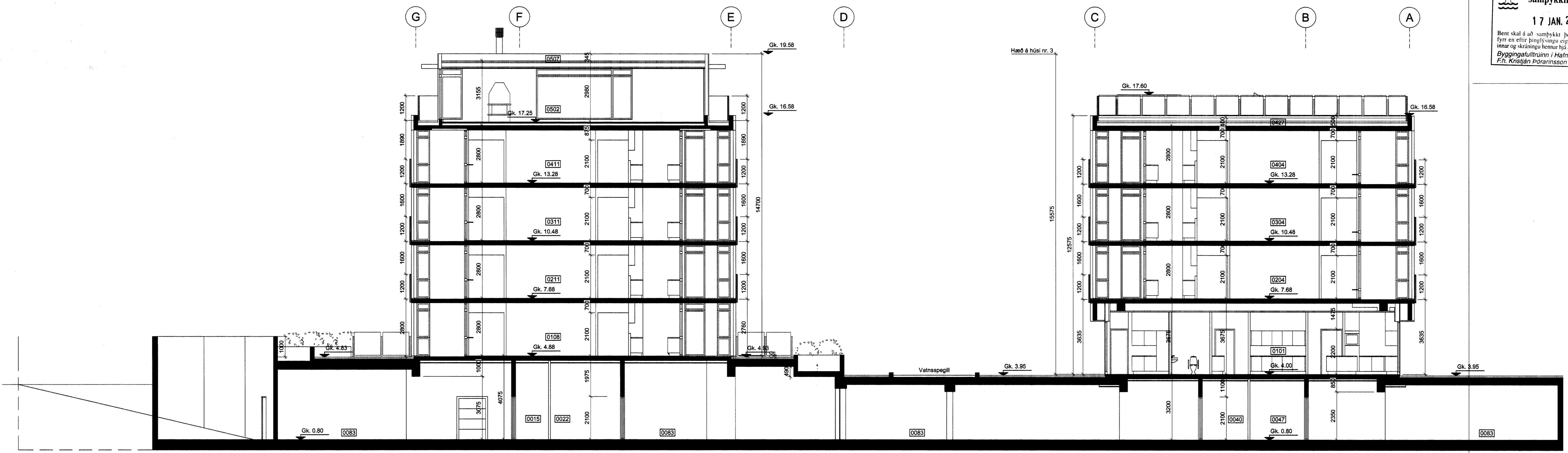
Þversnið A-A í húsi nr. 3
