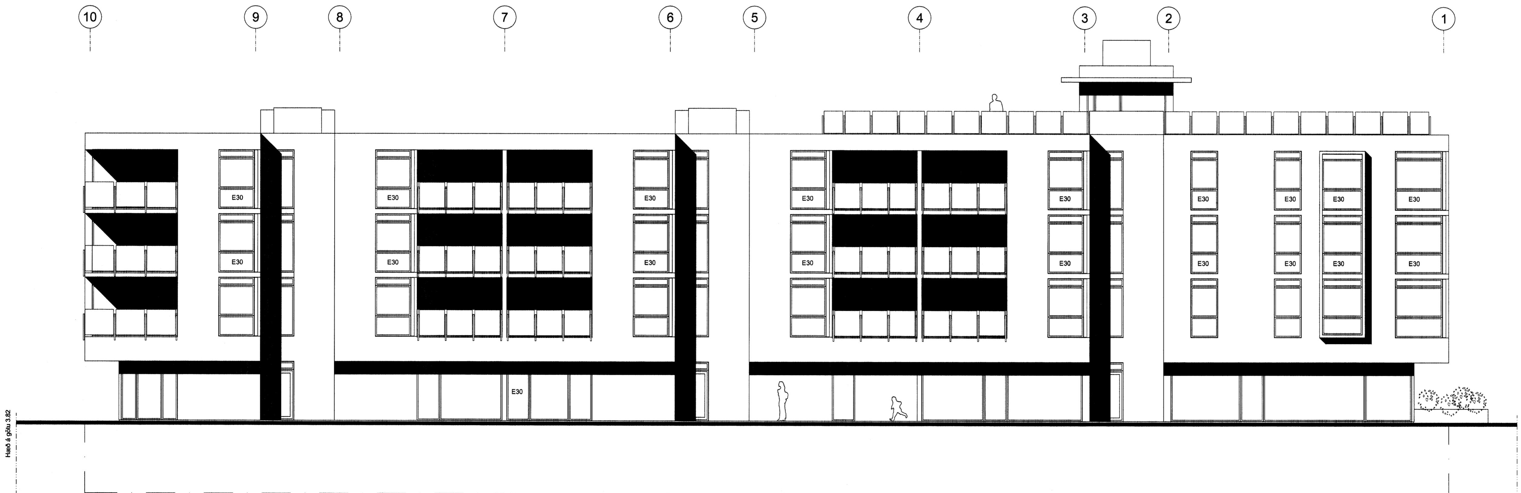
Norðurbakki 1 útlit Vestur
