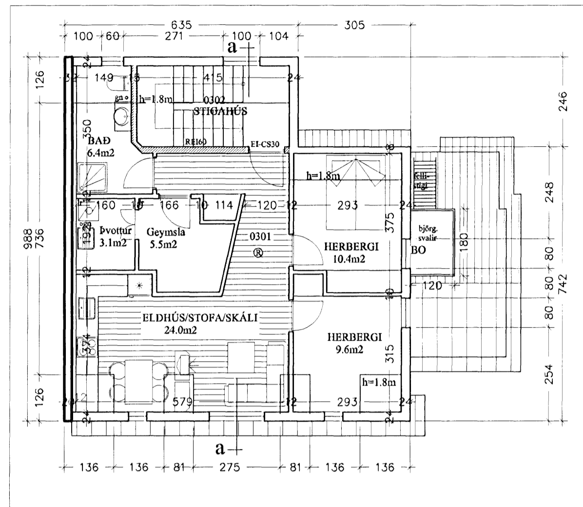
Grunnmynd 1.hæð 1:100
