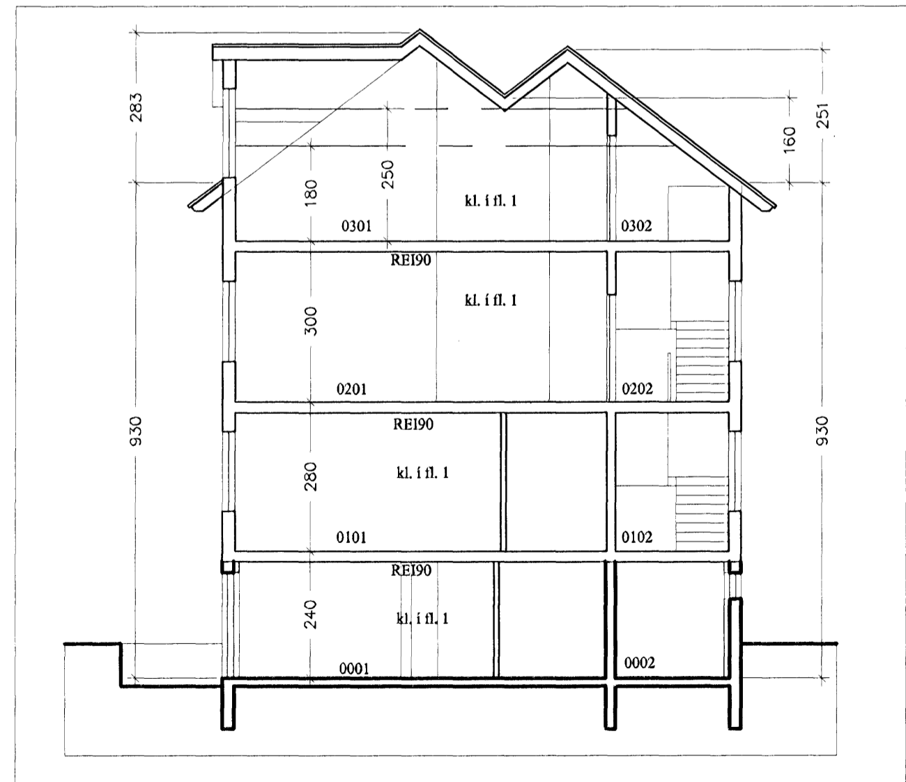
Sneiðing a-a 1:100
