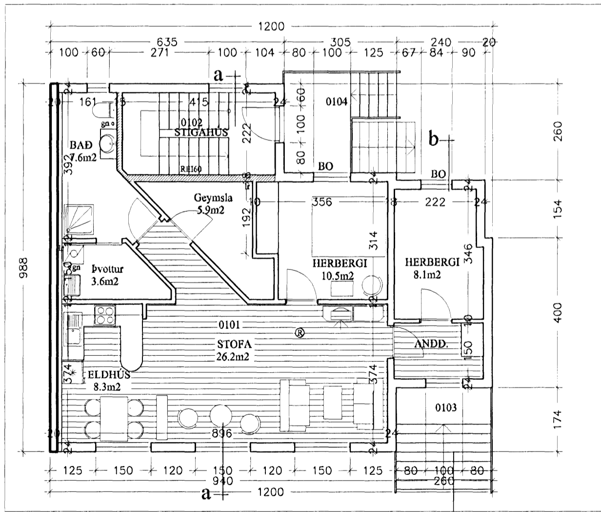
Grunnmynd 1.hæð 1:100
