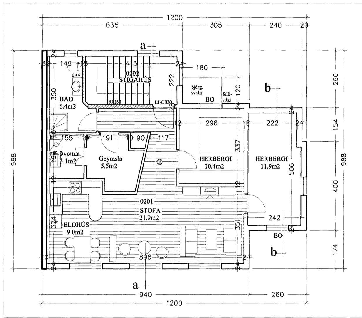
Grunnmynd 2.hæð 1:100
